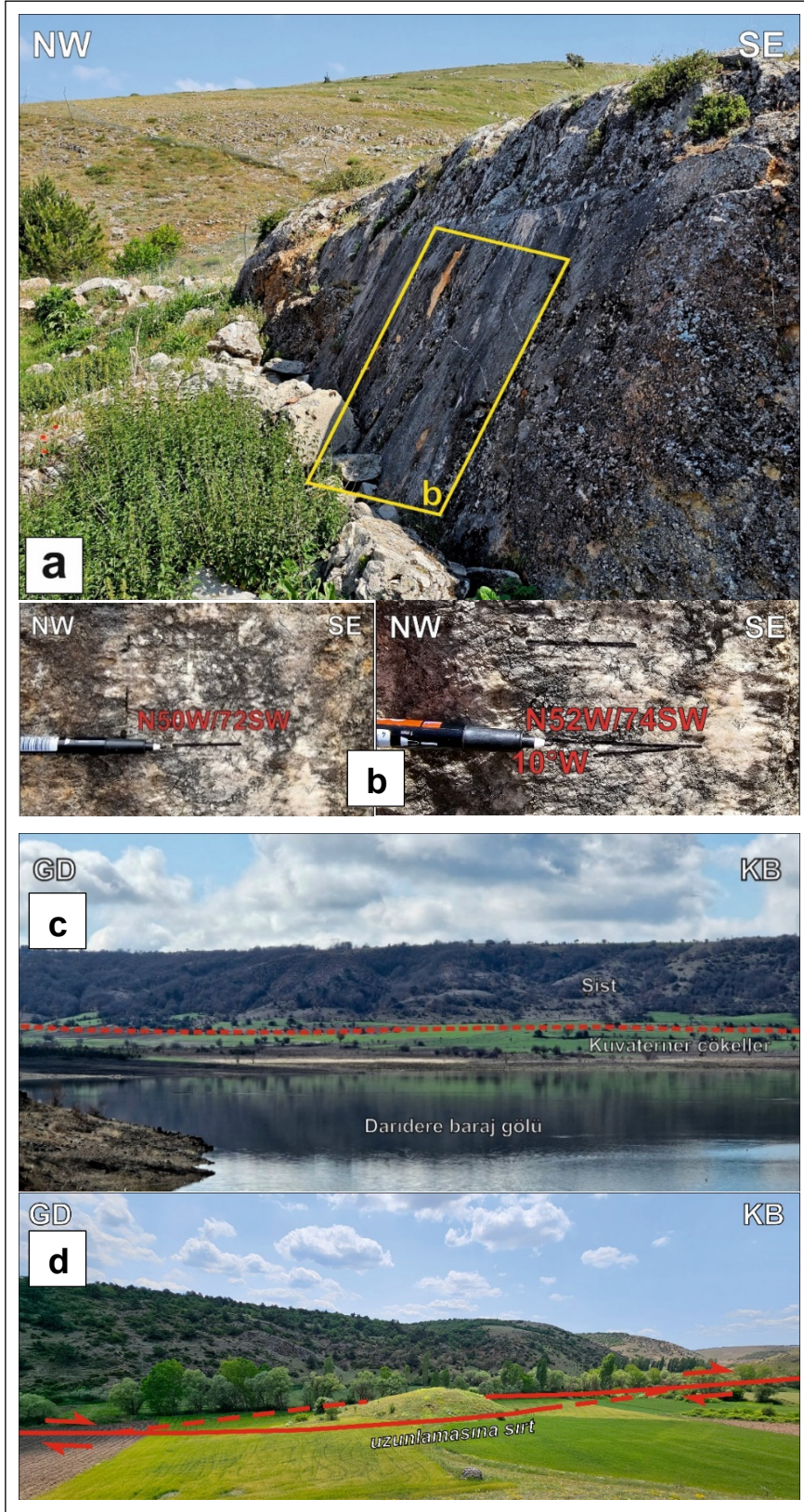
Şekil 4- Dodurga Fayı'nın 2 nolu segmenti boyunca a, b) Dodurga ilçesi güneydoğu girişinde ana kayadaki fay düzlemlerine örnekler, c) segment-2 kuzeybatısında Darıdere Barajı civarındaki temel birimler ile Holosen çökeller arasındaki yapısal sınırı ve d) Erenköy Mahallesi güneydoğusunda Dodurga Fayı boyunca gelişmiş uzunlamasına sırt yapısı.
