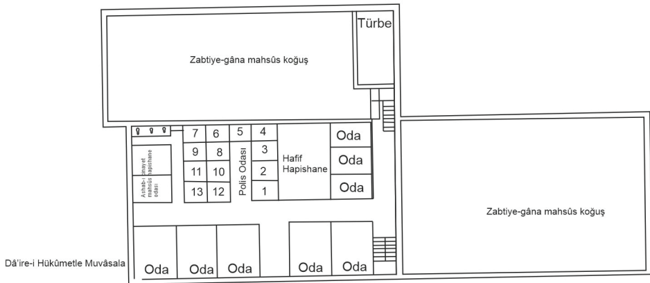
Çizim 3: 2. Kat Hapishane/Polis ve Zaptiye Birimlerinin Yer Aldığı Üst Kat Planı
