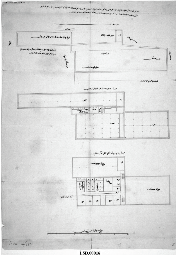
Fotoğraf 2: Erzurum Hapishanesi Plan Şemalarının Genel Görüntüsü (BOA. İŞD. 16/681. 005)
