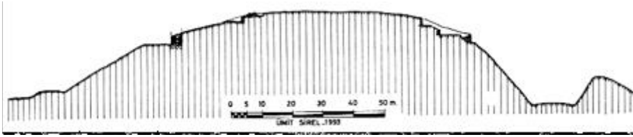
Çizim 2 Aşağı Anzaf Kalesi'nin kuzey-güney kesiti.
