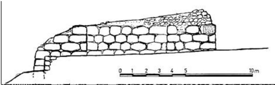
Çizim 11 Haldi Tapınağı doğu duvarı.
