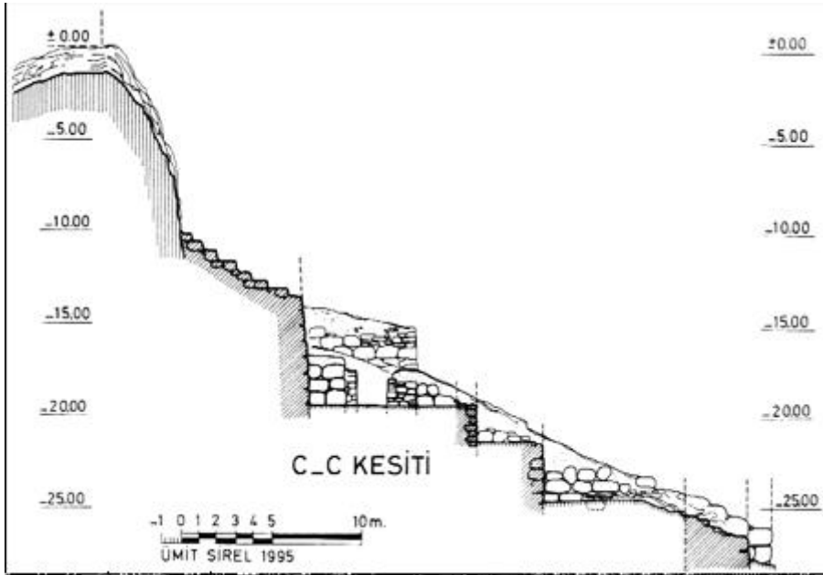
Çizim 9 Büyük kule, kuzey kapısı ve depo yapılarının kesiti.
