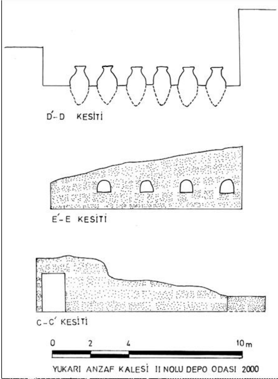
Çizim 16 II no'lu pithoslu depo odasının kesiti.
