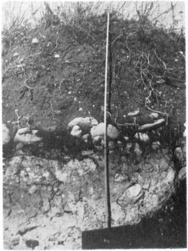
Foto 1 : Erzurum Ovası'nın kuzeybatısında Daphan Ovası'nda çakıllı, killi ve marnlı Pliyo-kuvaterner çökelleri üzerinde gelişmiş kahverengi toprak profili.
