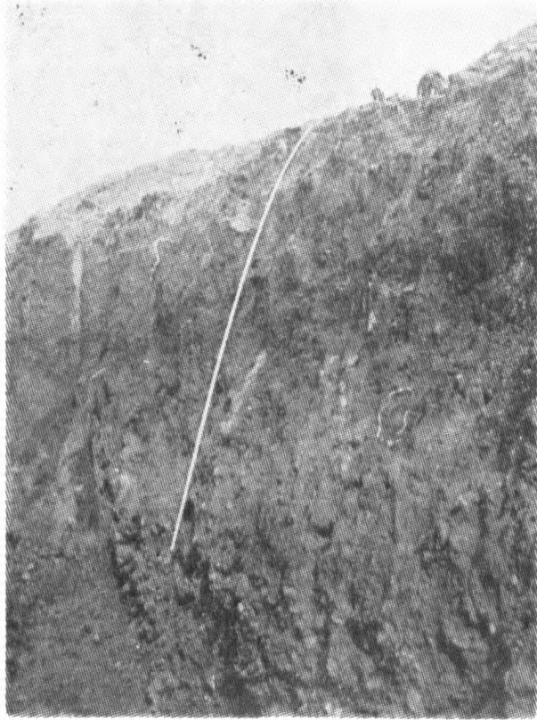
Foto 3 : Erzurum Ovası'nın güneyinde eski birikinti yelpazesini üzerinde oluşmuş kahverengi toprak profili.
