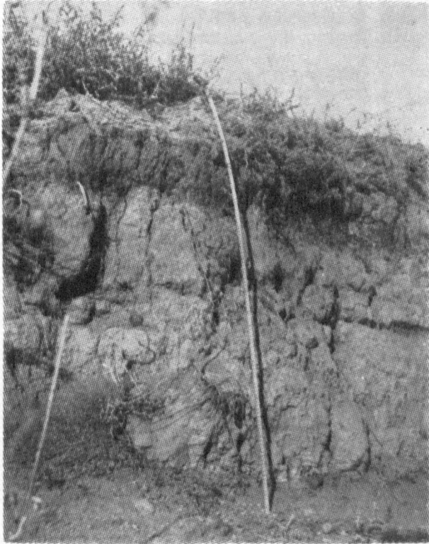
Foto 6 : Karasu Tivnik Köprüsü'nün doğusundaki alüvyial toprak profili, profildeki koyu renkli horizon organik madde bakımından zengindir. Photo 6 : An alluvial soil profile on just the east of Tivnik bridge, the dark horizon is rich in organic content.
