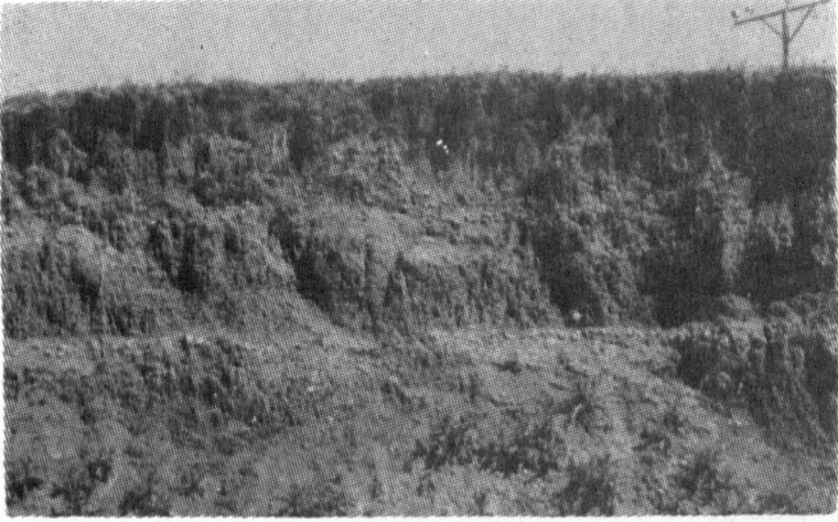
Foto 5 : Erzurum Ovası'nın batısında 1800 m yükseklikte çakıllı seviyeler gösteren yarı olgun kahverengi toprak profili. Photo 5 : The sub-mature brown soil containing gravelly horizon, on the western section of the Erzurum Plain.
