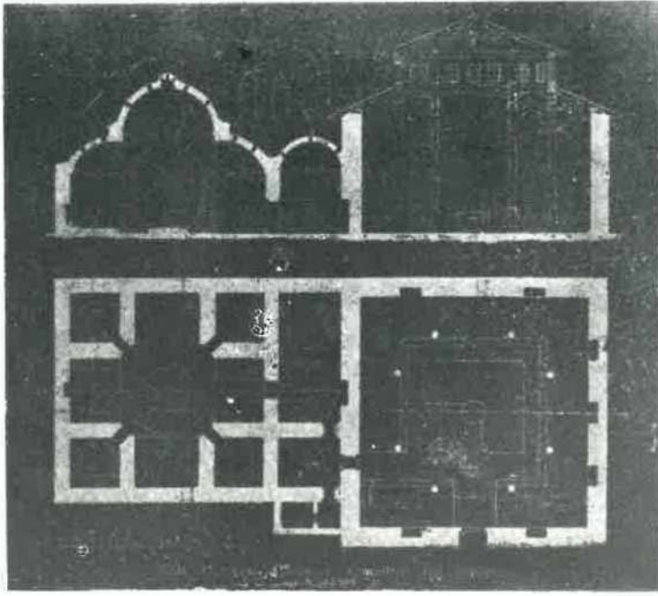
19 — Samatyada Ağa hamamı plân ve maktarı, H. g.
