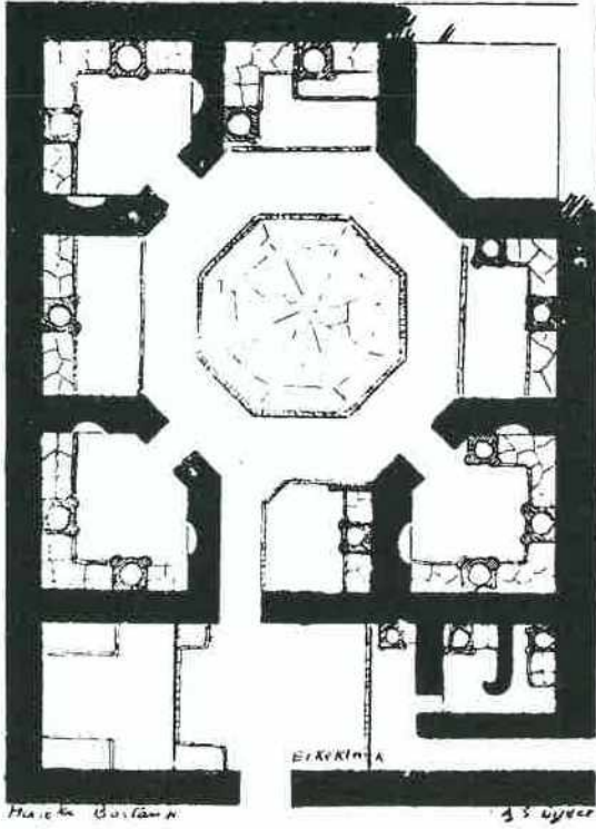
11 — Hasekide Bostan hamamı erkekler tarafı takribî plânı. (1921 de Dr. A. S. Ünver)
