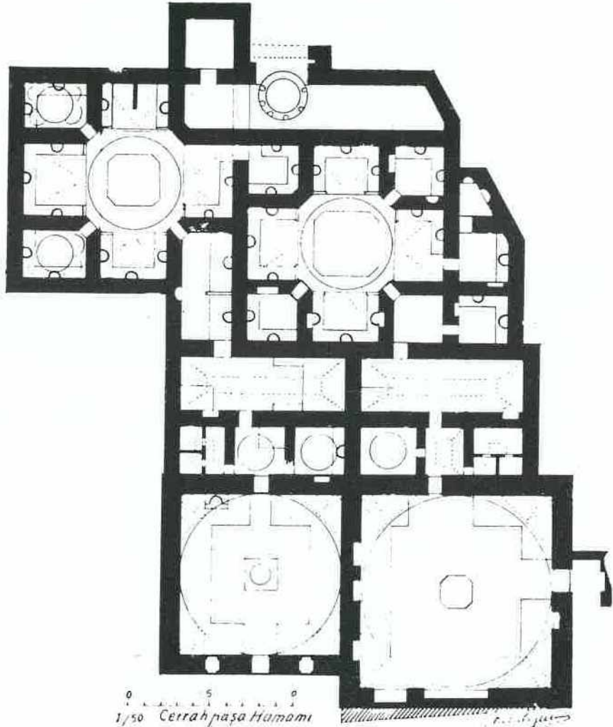
5 — Cerrahpaşa hamamı plânı. Elyevm bu hamam mevcut değildir. Mahallinde B. Münif Benli ile tarafımızdan aslına mütâbık bir surette 1/50 eb'adında çizilmiştir. 1931
