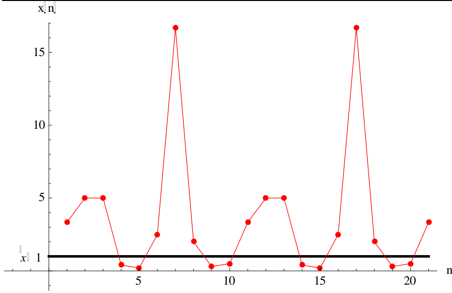
Şekil 9. x(n) çözümlerinin grafiği
