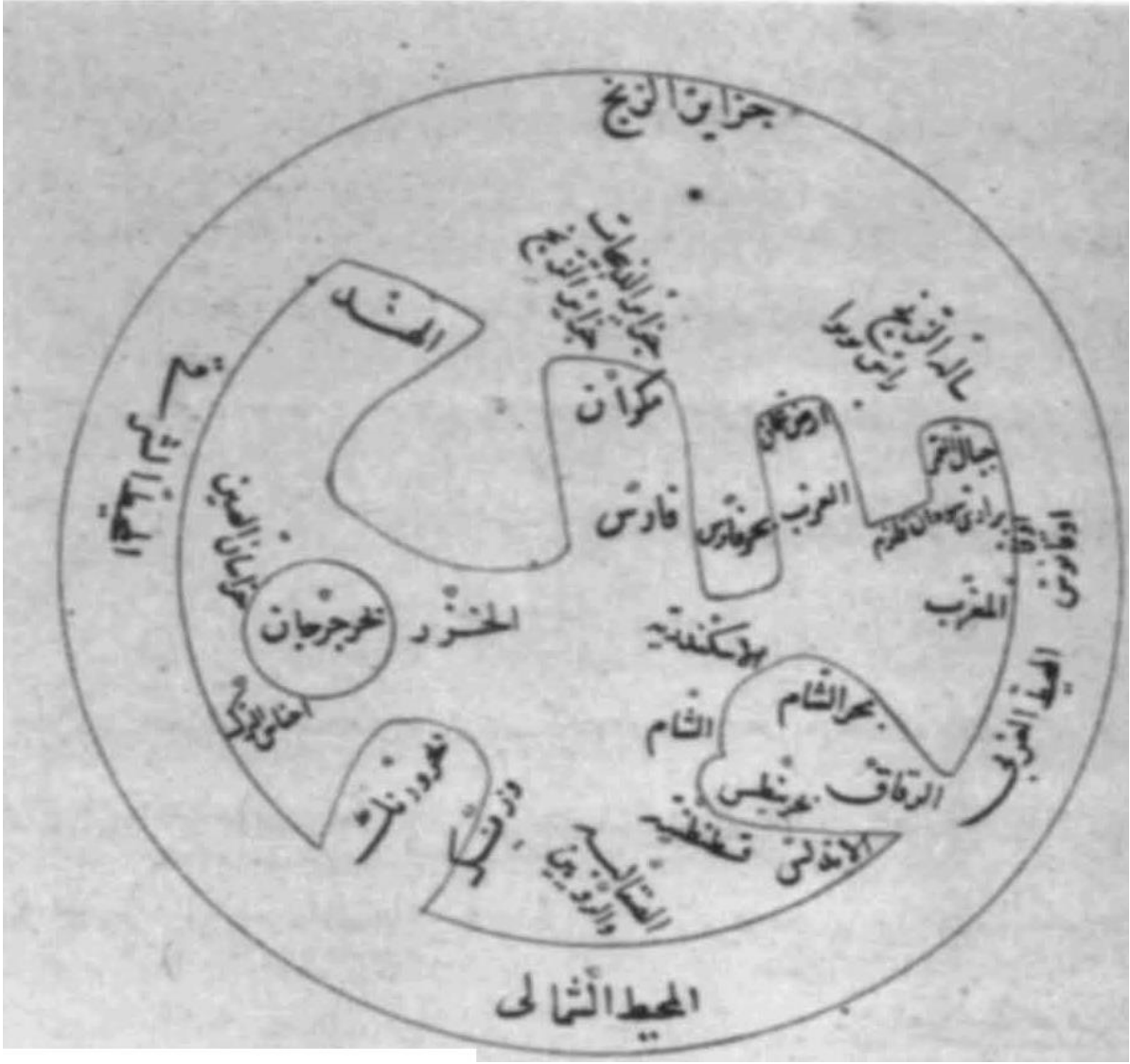
Birûnî'nin et-Tefhim adlı eserinden kara ve denizlerin dağılışına ait kroki (telif 420/1021)
