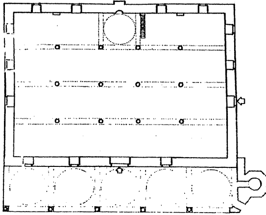
Bornova Büyük Câmi Plân Şeması 14
