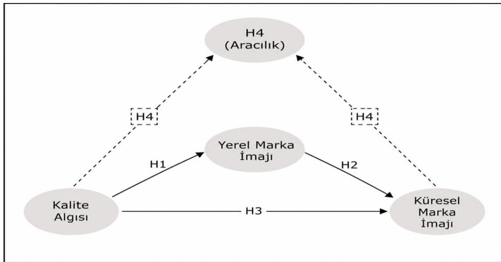
Şekil 1. Teorik Model
