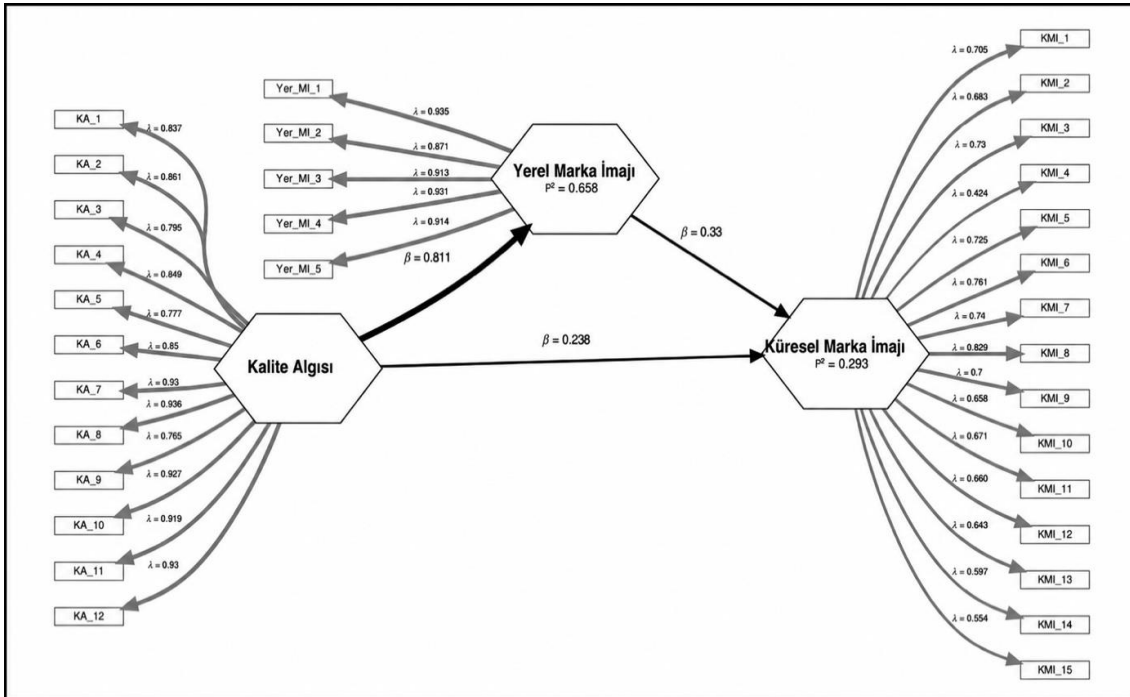
Şekil 2. Yol Modeli
