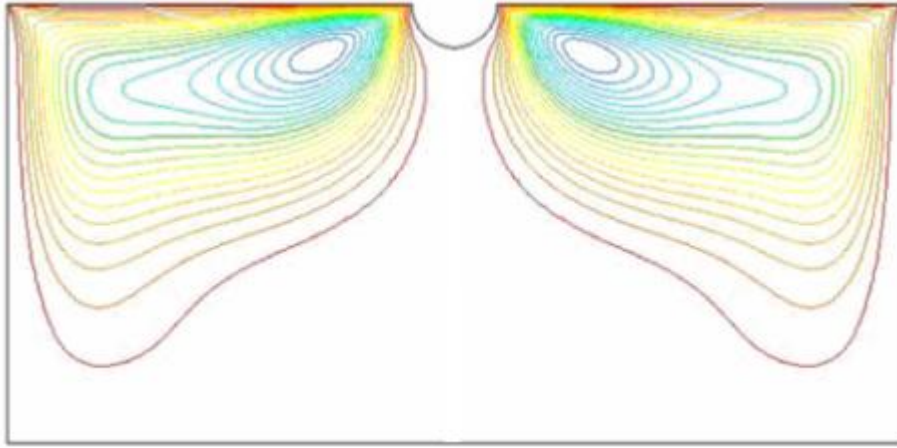
Şekil 6. Dikdörtgenler prizması şeklindeki konfigürasyon içerisinde kararlı yüzey gerilim konveksiyon hareketi yapan akışkanın akım hatları ( T_C= + 15 °C, T_H= + 40 °C ve T_R= + 23 °C) (Kati, 2009)
