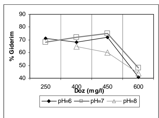
Şekil 10. \text{Al}_2(\text{SO}_4)_3 \cdot 18\text{H}_2\text{O} koagülantı ile AKM Giderimi.
