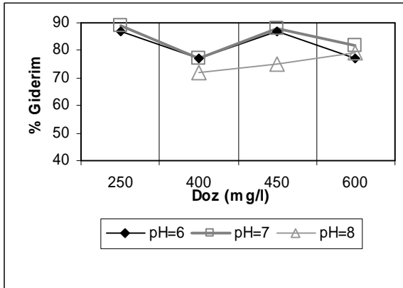
Şekil 9 \text{Al}_2(\text{SO}_4)_3 \cdot 18\text{H}_2\text{O} koagülantı ile KOI Giderimi.
