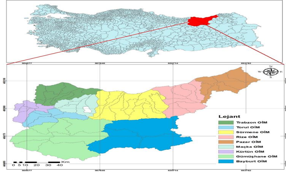
Şekil 1. Çalışma alanının lokasyon haritası
