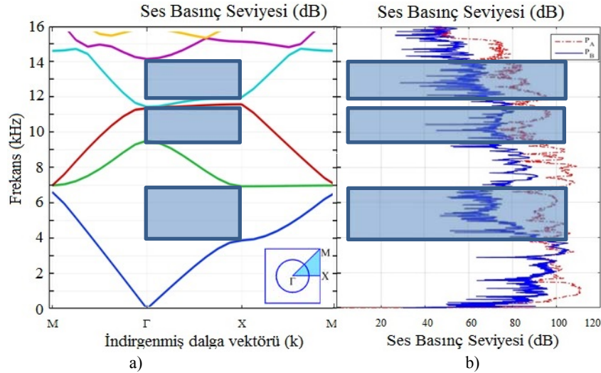
Şekil 3. a) Kare örgü bant yapısı b) deneysel olarak elde edilen ses basınç seviyesi [Sound Pressure Level (dB)] değeri
