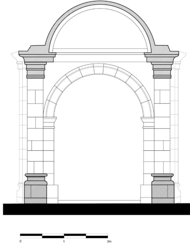
Çizim 1: Mustafa Zühtü Efendi Türbesi Kesiti
