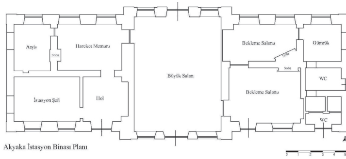
Şekil 02: Akyaka İstasyonu/Kat Planı
