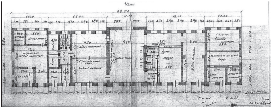
Şekil 04: Kars Eski İstasyon Binası Planı (1941) (TCDD Genel Müdürlüğü Arşivi)
