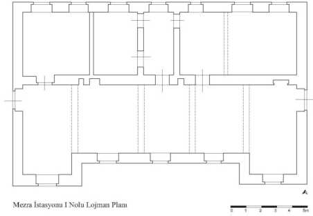
Şekil 05: Mezra İstasyonu/ 1 Nolu Lojman Binası Planı
