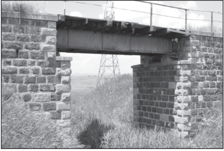
Resim 03: Doğukapı-Demiryolu Sınır Köprüsü
