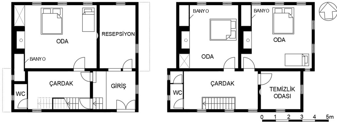
Zemin kat planı
