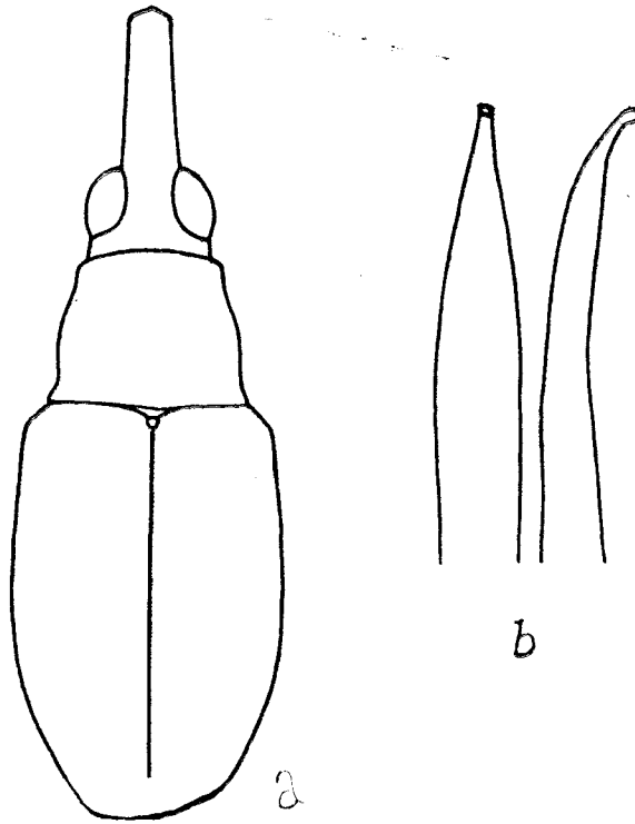
Fig. a-b; Apion subconsors n. sp. ♂ a: Umriss des Körpers- b: Aedaeagus.
