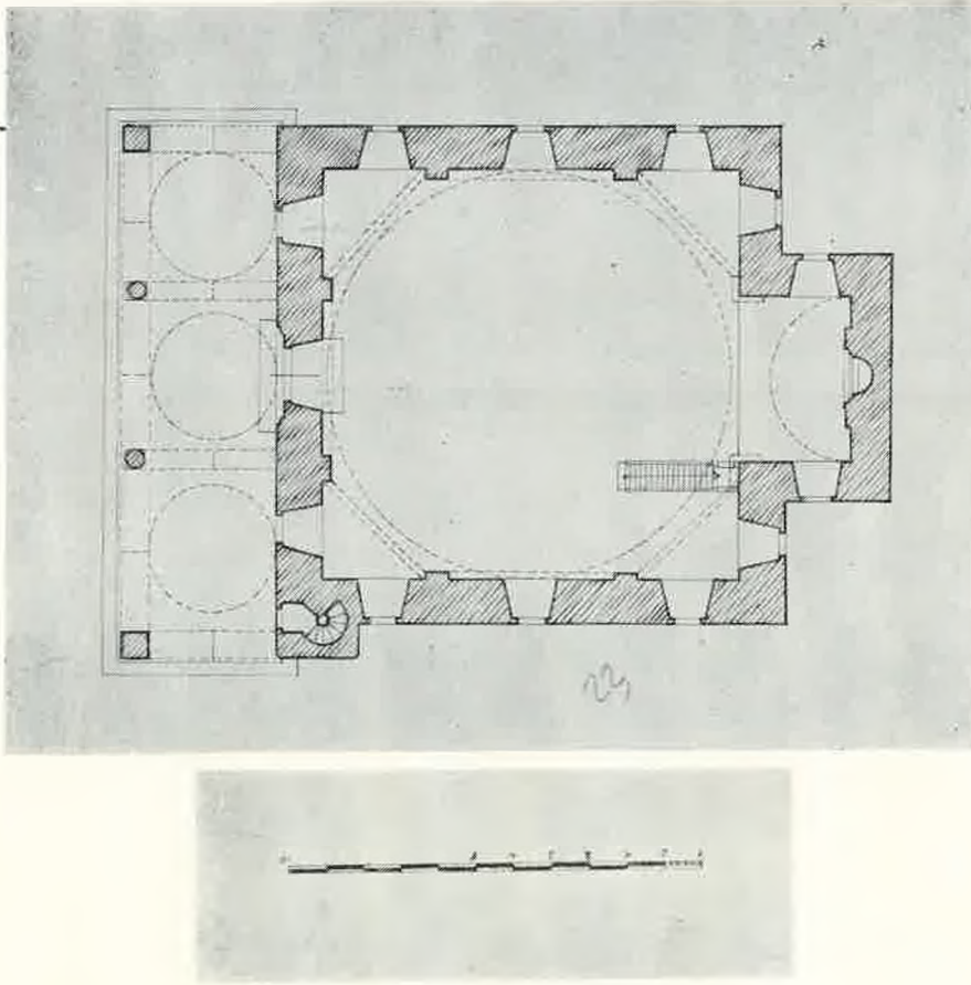
Resim : 1 — Şerefli Koçhisar Alâüddin camii plânı.
