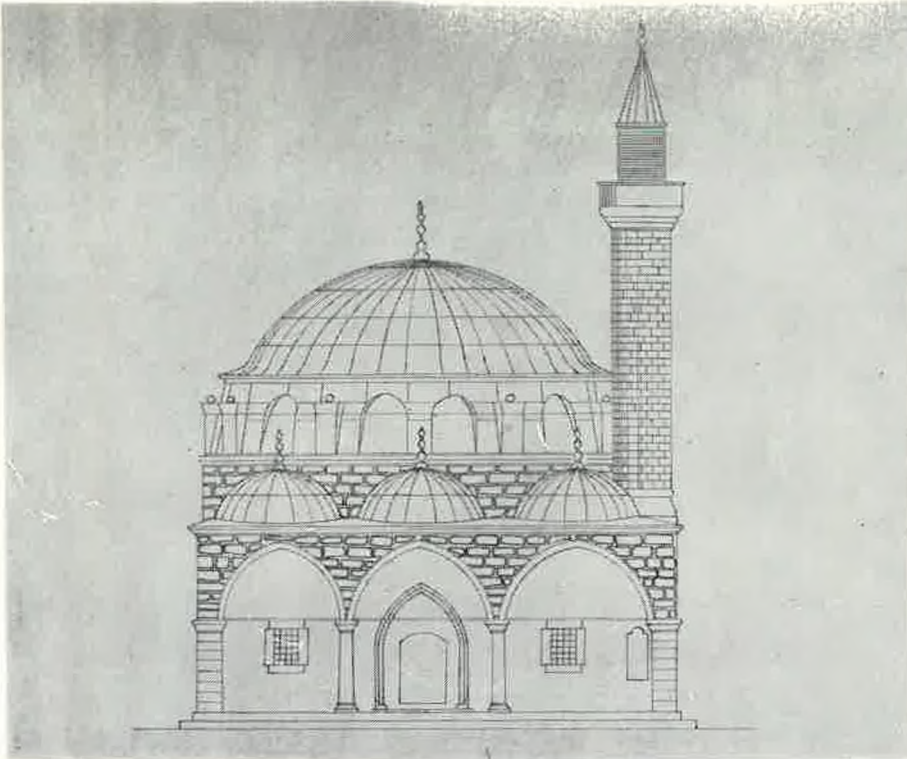
Resim : 2 — Camiin ön cephesi.
