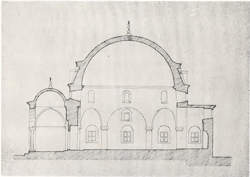
Resim : 4 — Camiin uzunlamasına kesiti.
