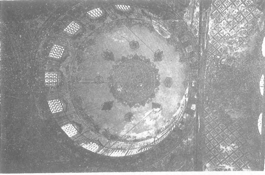
Resim 14 — Muradiye Camii kubbesinin iç görünüşü (Onarımdan önce)
