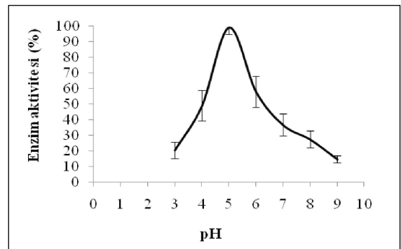
Şekil 5. pH'nin enzim aktivitesi üzerine etkisi Figure 5. Effect of pH on the enzyme activity
