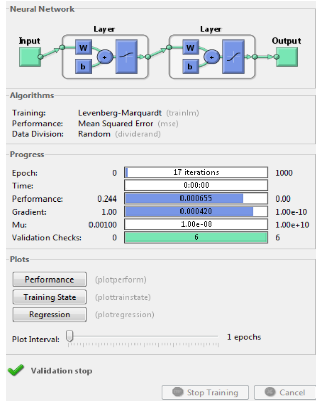
Şekil 6. YSA ile ağın eğitilmesi
