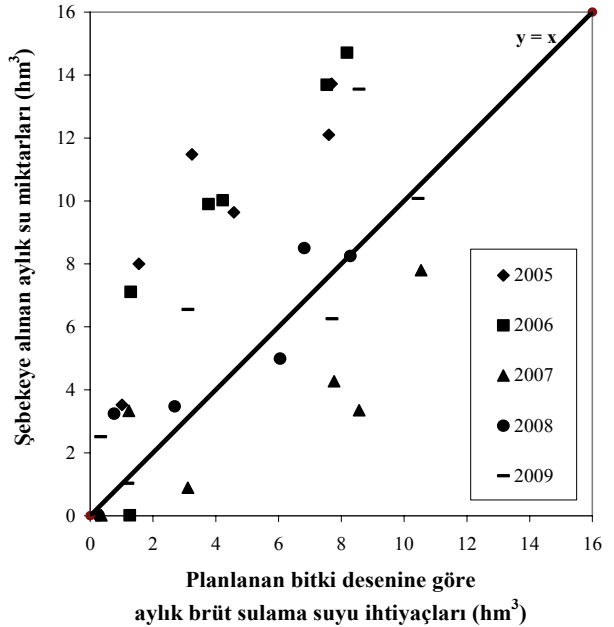
Şekil 4. Balıkesir Ovası 2005-2009 yılları planlanan bitki desenine göre aylık brüt sulama suyu ihtiyaçları ve şebekeye alınan aylık su miktarları arasındaki ilişki (Relation between monthly water taken to the network and monthly gross irrigation water needs according to planned plant pattern of Balıkesir Plain between the years 2005-2009)
