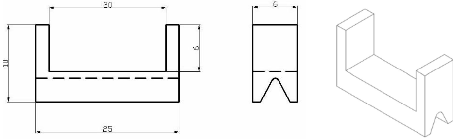
Şekil 4. Diş diplerinden tel erozyon yöntemi ile kesilerek elde edilen Deney numunesi
