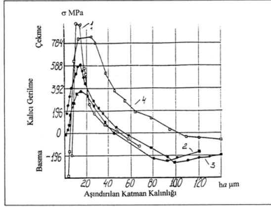
Şekil 1. Adımı 5mm, vida diş dibi yarıçapı r=0,508 mm olan çelik malzemeye açılmış vidaların diş diplerinde oluşan kalıcı gerilmeler \sigma_0 ; 1*. V=0,97 m/s; 2*. V=1,53 m/s; 3*. V=2,43 m/sn; 4**. V=1,53 m/s * Kesme sıvısı kullanılmış ** Kesme sıvısı kullanılmamış
