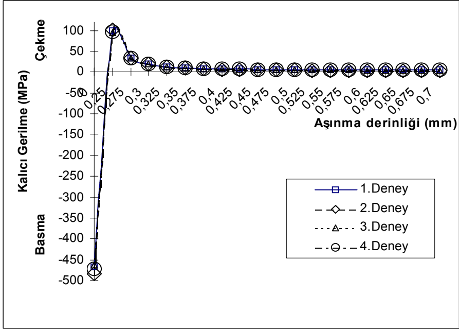
Şekil 6. AISI 5115 çelikten imal edilen ve semantasyon işlemi uygulanmış bir dişli çarkın diş dibinde oluşan kalıcı gerilme dağılımı
