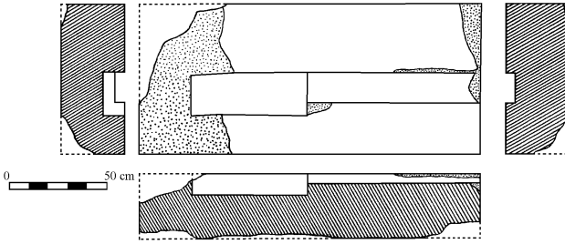
Fig. 5 İkiiztepe Tümülüsü 1 no.lu altlık çizimi.
