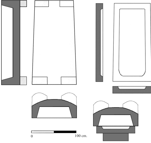
Fig. 12 İkiiztepe Tümlüsü kapaklı kline çizimi. Özgen - Öztürk 1996, Fig. 98
