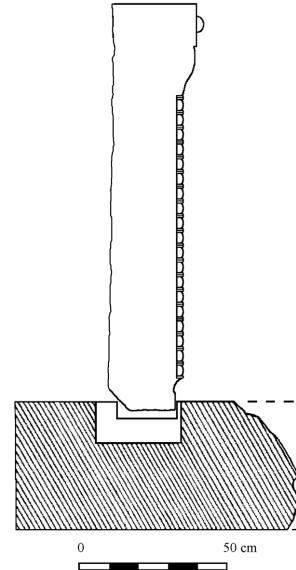
Fig. 11 İkiiztepe Tümülüsü, kapı steli-altlık çizimi.
