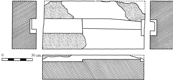
Fig. 6 İkiiztepe Tümülüsü 2 no.lu altlık çizimi.
