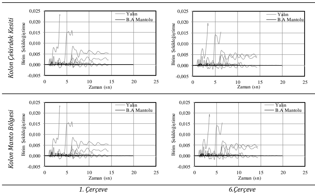
Şekil 17. Şekildeğiştirme geçmişi
