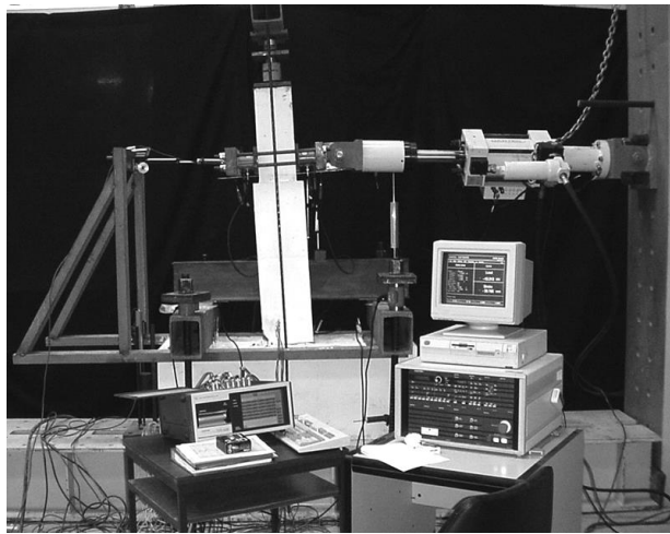
Şekil 2. Deneysel düzeneği [17]
