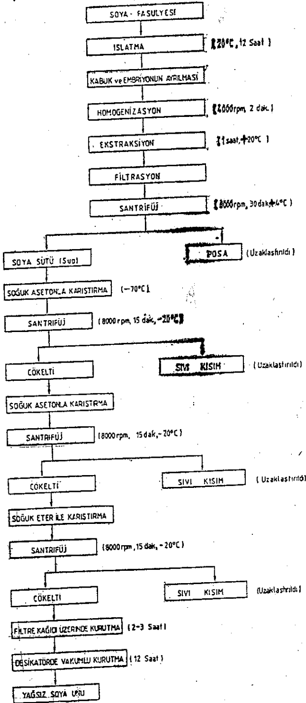
Şekil 1: Yağsız Soya Unu Üretimi (NAKAMURA ve Ark., 1986).
