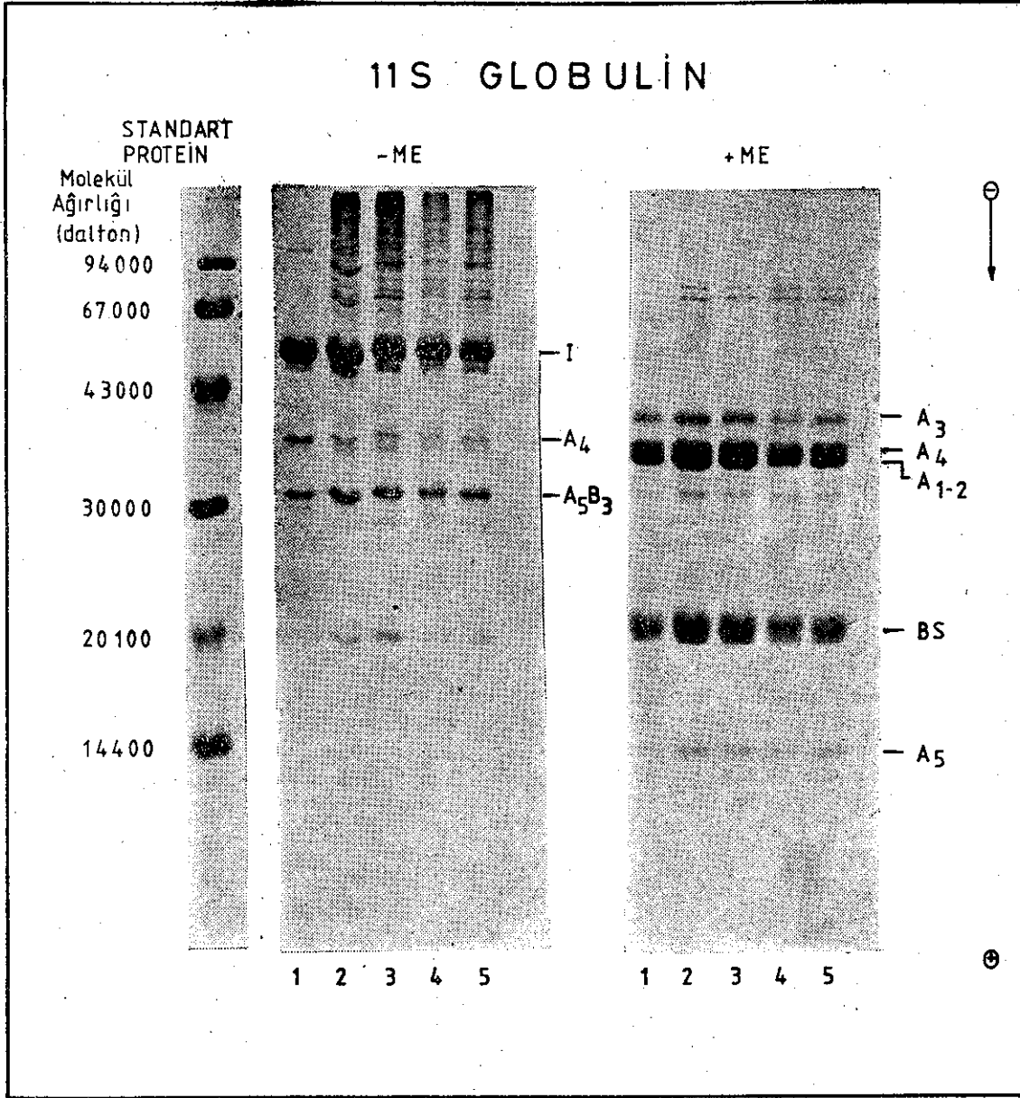
Şekil 4 : Türkiye'de yetiştirilen bazı soya varyetelerinin 11S globulin fraksiyonlarının SDS-PAGE analizi, 1: IOR, 2: ALTONA, 3: CORSOY, 4: CALLAND ve 5: BEASON.
