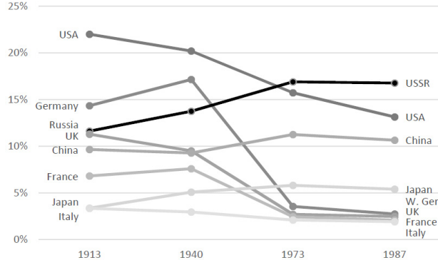
Şekil 2. Uluslararası sistemdeki büyük güçler, 1913'den 1987'ye (seçili yıllar) ulusal kapasite birleşik endeksi
