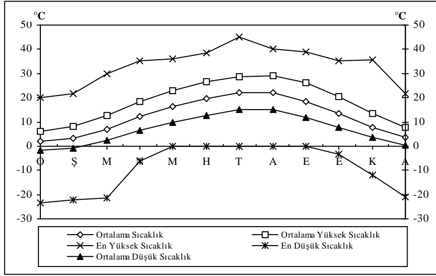
Şekil 2. Tokat'ta Sıcaklık Değerlerinin Aylık Ortamaları (1930-2003)
