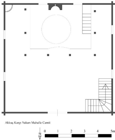
Çizim 9- Kargı Yukarı Mahalle Camii Planı Resim 9- Gürgenliyatak Mahallesi Merkez Camii İç Mekânı
