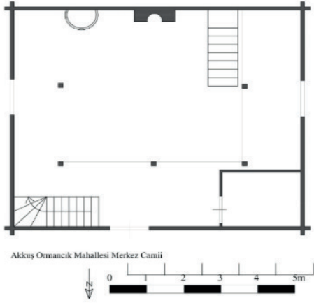
Çizim 4- Ormancık Mahallesi Merkez Camii Planı Resim 4- Ormancık Mahallesi Merkez Camii'nin Eski Hali
