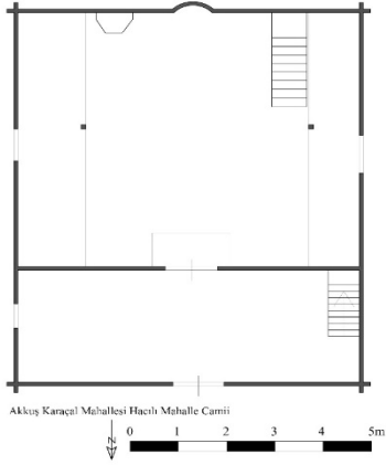
Çizim 2- Karaçal Mahallesi Hacı Mahalle Camii Planı Resim 2- Karaçal Mahallesi Hacı Mahalle Camii Görünüşü
