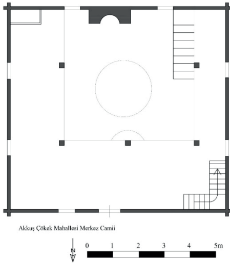
Çizim 6- Çökek Mahallesi Merkez Camii Planı Resim 6- Ambargürgen Mahallesi Merkez Camii Görünüşü
