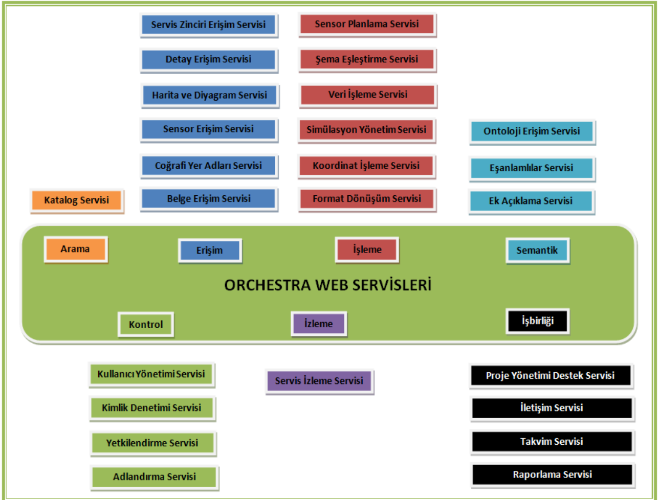
Şekil 4. ORCHESTRA web servisleri için fonksiyonel sınıflandırma ([32]'den esinlenerek üretilmiştir).
