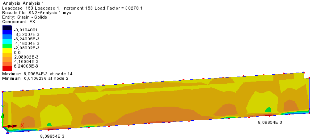
Şekil 21: SN2 deney kirişine ait LP'nin analiz sonucu şekil değiştirme dağılımı
