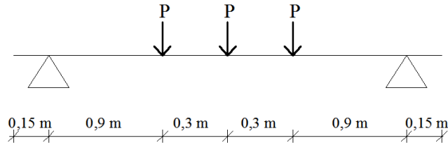
Şekil 12: Moment taşıma gücünden yük tayini
