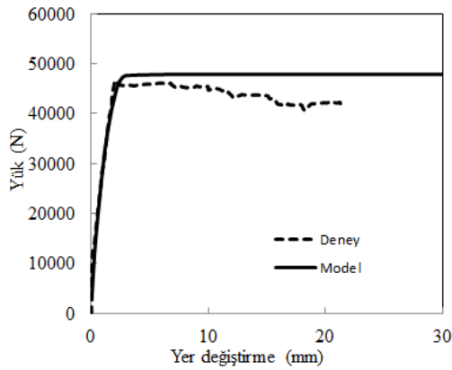
Şekil 17: a. KN deney kirişine ait yük-yer değiştirme ilişkisi b. Deneysel sonrası kirişin görünüşü
