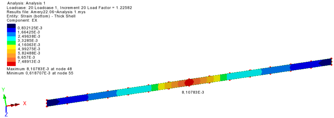
Şekil 9: RR3 deney kirişine ait LP'nin DP kriteri ile analiz sonucu şekil değiştirme dağılımı
