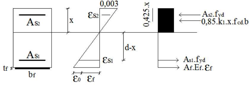
Şekil 11: LP ile güçlendirilmiş kirişte iç kuvvet denge durumu
