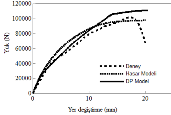
Şekil 8: RR3 kirişine ait yük-yer değiştirme ilişkisi
