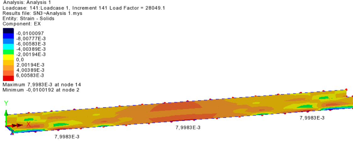
Şekil 23: SN3 deney kirişine ait LP'nin analiz sonucu şekil değiştirme dağılımı
