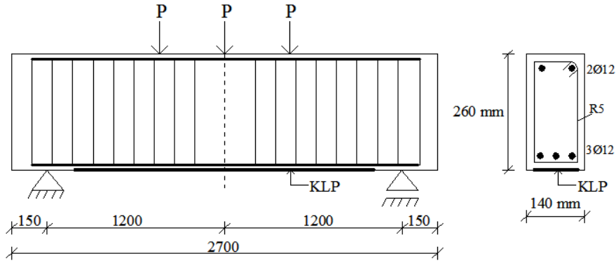
Şekil 6: RR3 kiriş geometrisi ve donatı düzeni (Al-Amery and Al-Mahaidi, 2006)
