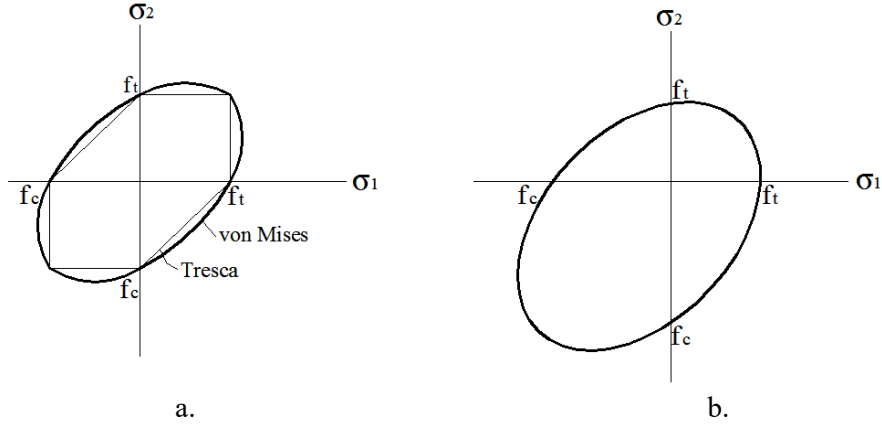
Şekil 5: a. von-Mises, b. geliştirilmiş von-Mises akma kriteri
