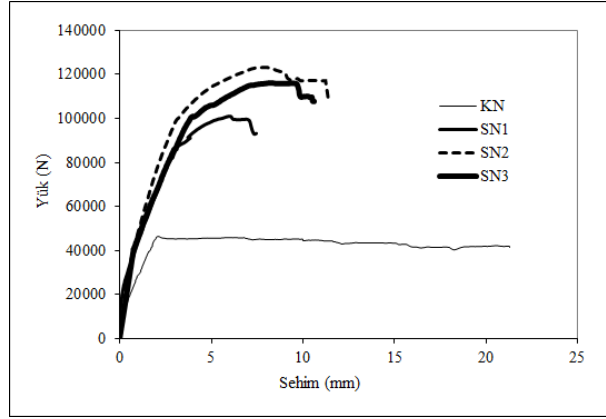
Şekil 15: Deneysel kirişlerin karşılaştırmalı yük sehim grafiği (Köksal ve diğ., 2017)
