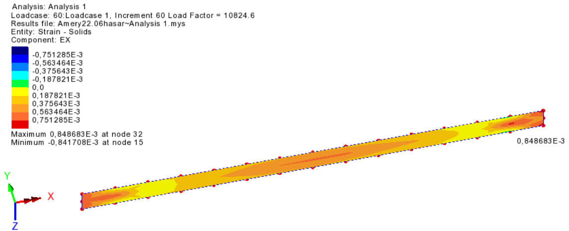
Şekil 10: RR3 deney kirişine ait LP'nin hasar modeli ile analiz sonucu şekil değiştirme dağılımı
