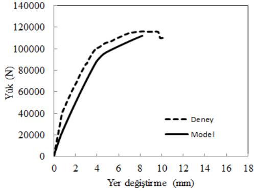
Şekil 24: a. SN3 deney kirişine ait yük-yer değiştirme ilişkisi b. Deney sonrası kirişin görünüşü
