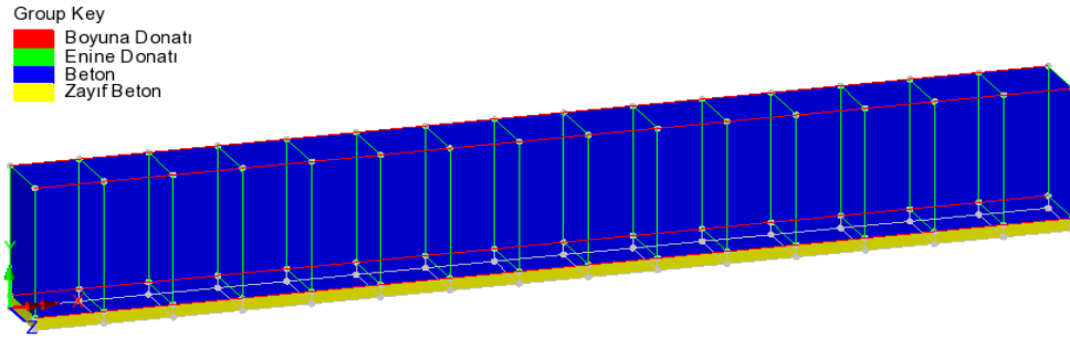
Şekil 16: KN deney kirişinin numerik modeli
