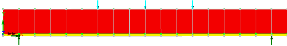
Şekil 7: RR3 kirişine ait oluşturulan sonlu eleman modeli
