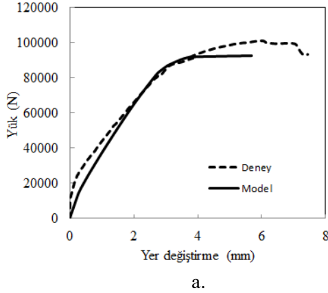
Şekil 19: a. SN1 deney kirişine ait yük-yer değiştirme ilişkisi b. Deney sonrası kirişin görünüşü
