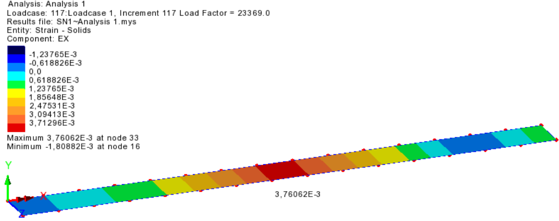
Şekil 18: SN1 deney kirişine ait LP’nin analiz sonucu şekil değiştirme dağılımı
