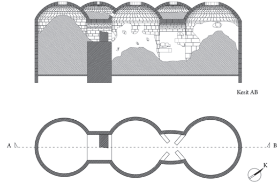
Fig. 9. D 6 Sarnıcı Kesiti, Termessos (Çizim: Y. Goubin)
