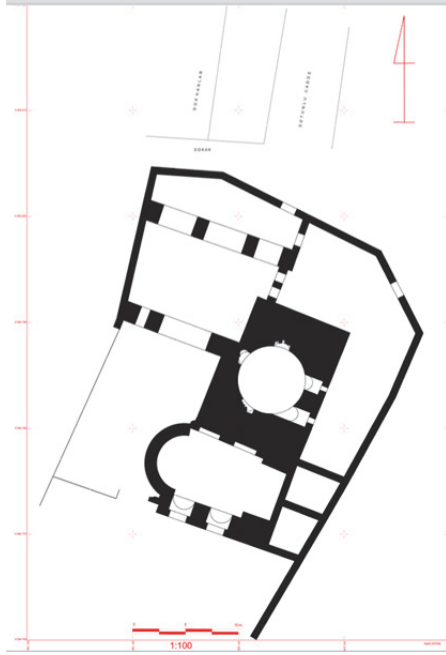
Fig. 10. Sütunlu Cadde Güneyindeki Yeni Hamam (Çizim: S. Aydal)
