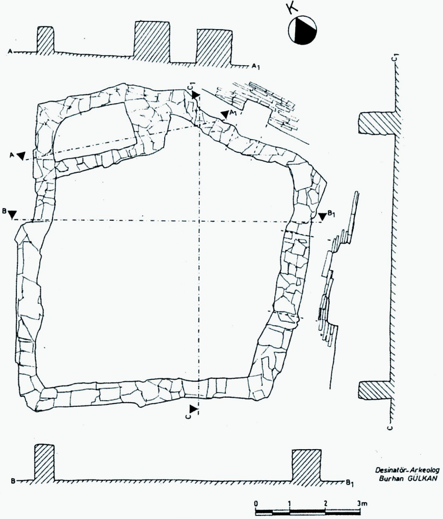
5. Açıma Yapısı Plan ve Kesiti BOYABAT - KOVUKLUKAYA
