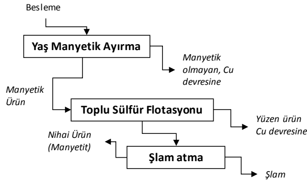
Şekil 6. d_{90}=75 \mu\text{m} ve d_{90}=53 \mu\text{m} 'a öğütülmüş numunelere uygulanan testlerin şematik görünümü. Figure 6. Schematic view of the tests applied to the samples ground to d_{90} = 75 \mu\text{m} .
