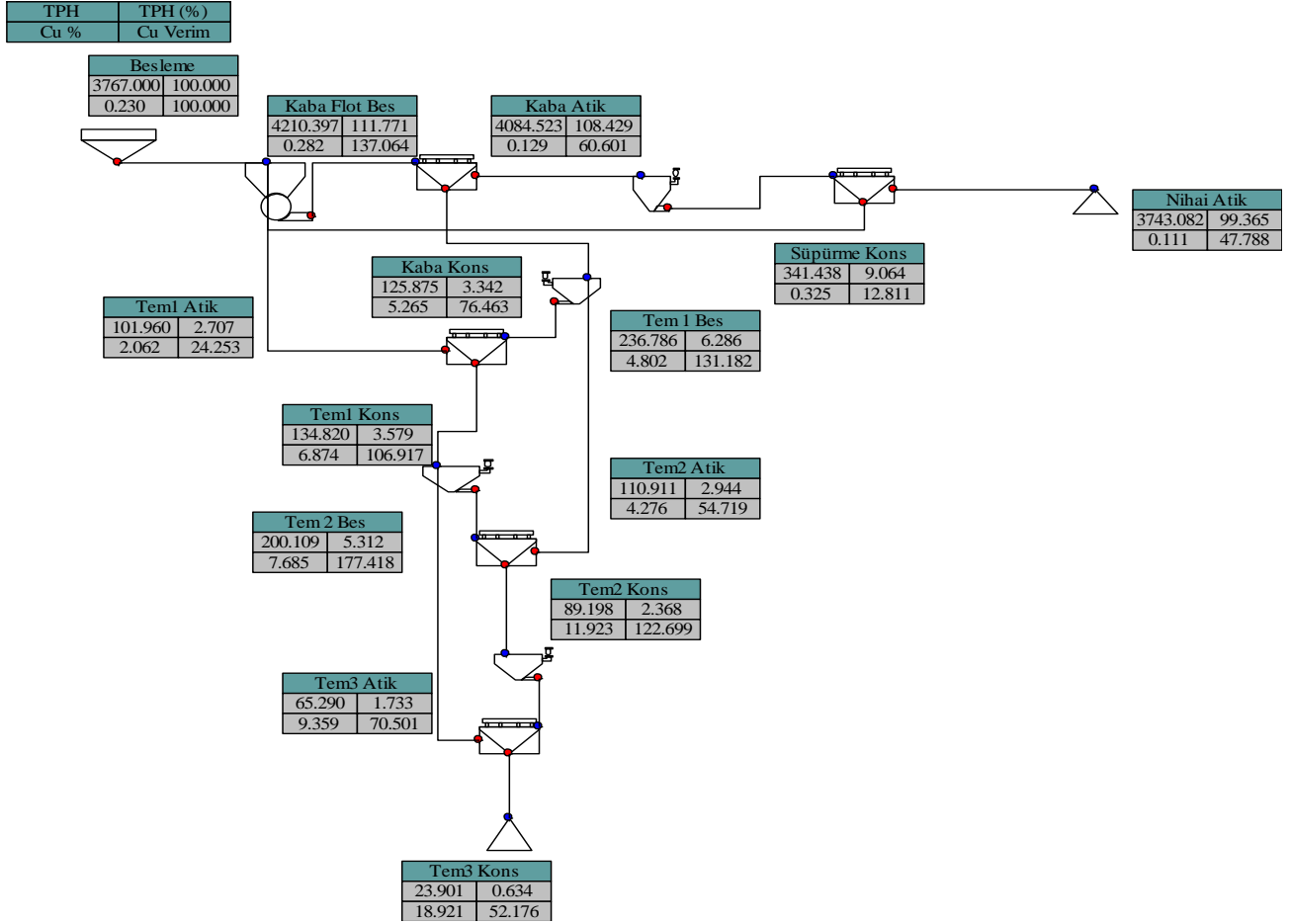
Şekil 15. Bakır flotasyon devresi simülasyon sonuçları.
