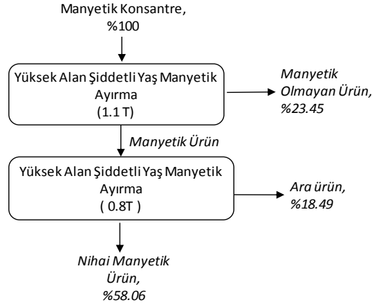
Şekil 13. Düşük alan şiddeti manyetik ayırma atığına uygulanan yüksek alan şiddetli manyetik ayırma işlemi sonucunda alınan ürünler.
