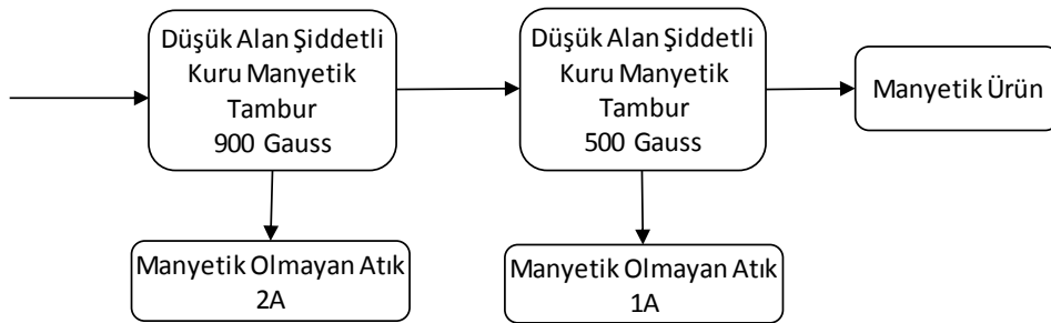
Şekil 3. -10 mm'ye kırılmış numune ile yapılan düşük alan şiddetli kuru manyetik ayırma (cobbing) testleri şematik görünümü.
