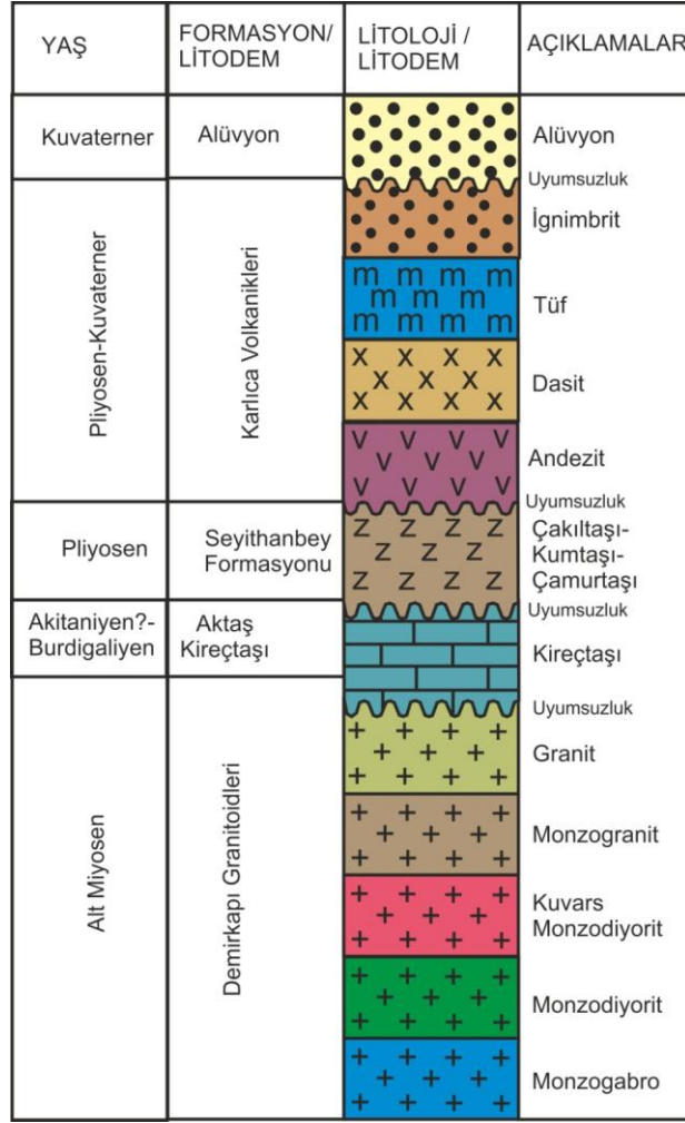
Şekil 2. Çalışma alanının genelleştirilmiş stratigrafik kesiti (ölçeksiz) (Davran, 2018).
