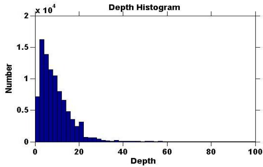
Figure 6. Earthquake-depth histogram. Şekil 6. Deprem-derinlik histogramı.
