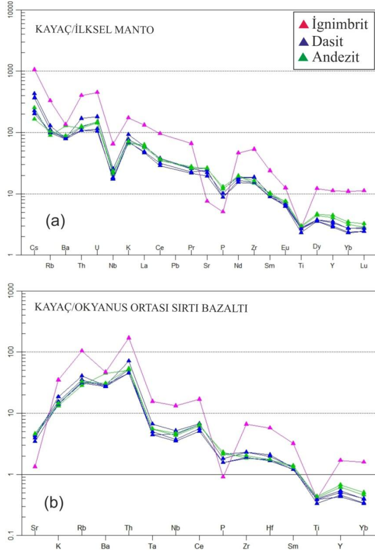
Şekil 6. Volkanik birimlerin a) Kayaç/İlksel Manto'ya göre normalize edilmiş eser element değişim diyagramı (Normalize değerleri Sun ve Mc Donough, 1989'dan alınmıştır) b) Kayaç/Okyanus Ortası Sırtı Bazaltı'na göre normalize edilmiş eser element değişim diyagramı (Normalize değerleri Pearce, 1983' den alınmıştır).
