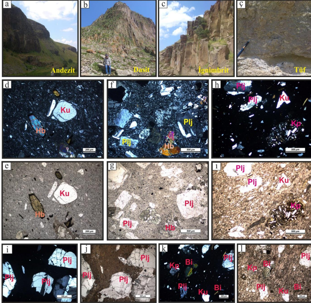
Şekil 3. Karlıca volkanitlerine ait arazi (a: Andezit; b: Dasit; c: İgnimbrit; ç: Tüf) ve polarizan mikroskop görüntüleri. d-e) Andezit (ÇN-TN); f-g) Dasit (ÇN-TN); h-i) İgnimbrit (ÇN-TN); i-j) Kristal tüf (ÇN-TN); k-l) Vitrik tüf (ÇN-TN). (Plj: plajiyoklaz, Hb: hornblend, Bi: biyotit, Ku: kuvars, Kp: kayaç parçası, ÇN: çift nikol, TN: tek nikol).
