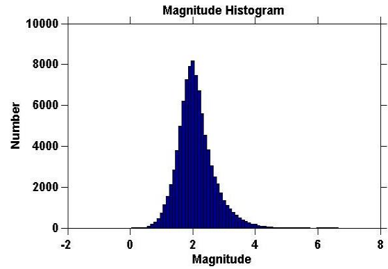
Figure 7. Earthquake-magnitude histogram. Şekil 7. Deprem-büyüklik histogramı.
