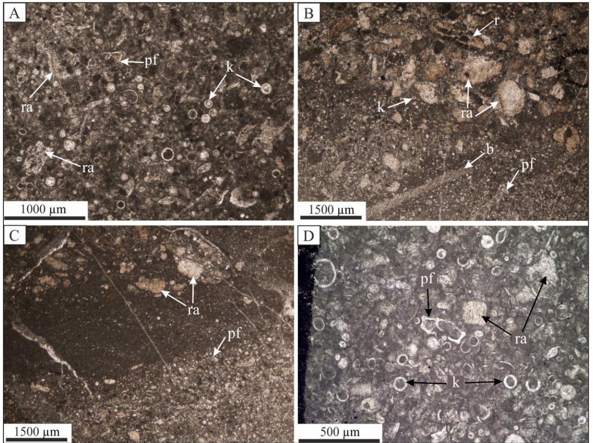
Şekil 7. D2 dolgusunun mikrofasiyes özelliklerini gösteren mikrofotograflar. A) D2 dolgusu tipik olarak seyrek planktonik foraminifer (pf), kalsisifer (k) ve rekristalize allokemler (ra) içeren Vaketaşı/Çamurtaşı dokusu ile temsil edilir (örnek no: 03-640). Planktonik foraminiferler baskın olarak dicarinellid ve marginotruncanid türleri ile temsil edilir. B) Rekristalize allokemlerin (ra) bolluğu bazı düzeylerde artar. Allokemlerin çoğunun biyoklastlara (b) ait olduğu anlaşılabilir. Bölümsel olarak rekristalize olmuş tanelerden bazılarının da rudist kavkı parçası (r) olduğu anlaşılabilir. Planktonik foraminifer (pf) ve kalsisiferlerin (k) bolluğu bazı örneklerde belirgin şekilde azalır (örnek no: 03-646), C) D2 dolgusunda bazı kesimlerde laminalanma gözlenir (pf: planktonik foraminifer, ra: rekristalize allokemler) (örnek no: 03-644), D) Bey Dağları Otoktonu'nun kuzey bölümünde gözlenen Koniasiyen-Santoniyen yaşlı yarıpelajik kireçtaşlarına ait tipik mikrofasiyes görüntüsü (örnek no: 03-142; Kocaboğaz Dere, Koordinat: 80820/47563). Fasiyes baskın olarak D2 dolgusunda olduğu gibi, tipik olarak seyrek planktonik foraminifer (pf), kalsisifer (k) ve rekristalize allokemler (ra) içeren Vaketaşı dokusu ile temsil edilir.
