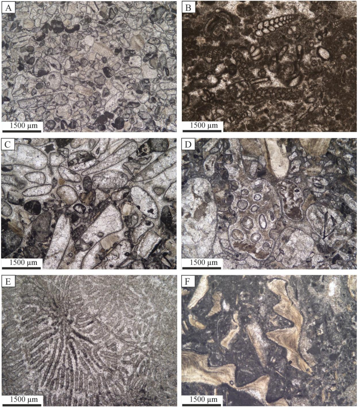
Şekil 5. Yan kayacı oluşturan platform kireçtaşlarında tanımlanan mikrofasiyes türlerine bazı örnekler. A) Yıkanmış biyoklastlı ve intraklastlı Tanetaşı mikrofasiyesi. Olasılıkla rudist ve mercan parçaları olan biyoklastlar çoğunlukla iyi yuvarlaklaşmış ve mikritik zarflarla sarılmıştır. Neredeyse tüm allokemler ve ilksel ortospar çimento yeniden kristalleşmiştir (örnek no: 03-608), B) Bol bentik foraminiferli ve seyrek intraklastlı Vaketaşı/İstiftaşı mikrofasiyesi (örnek no: 03-634), C) Yıkanmış biyoklastik Kabataş mikrofasiyesi. Dokusal özellikler A'ya benzer, ancak allokemlerin boyu belirgin şekilde daha büyüktür (örnek: 03-607), D) Biyoklastlı Tanetaşı/Kabataş
