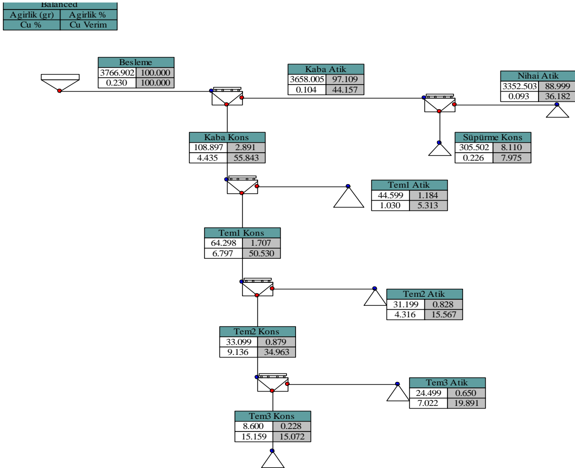
Şekil 14. Elde edilen en iyi bakır flotasyon devresi .
