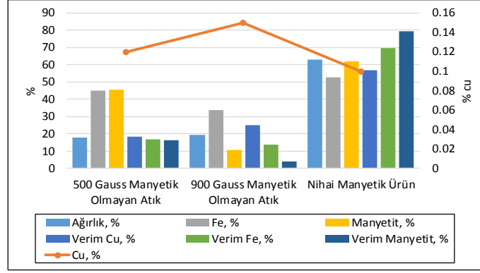
Şekil 7. Düşük alan şiddetli kuru manyetik tambur ürünlerinin özellikleri.
