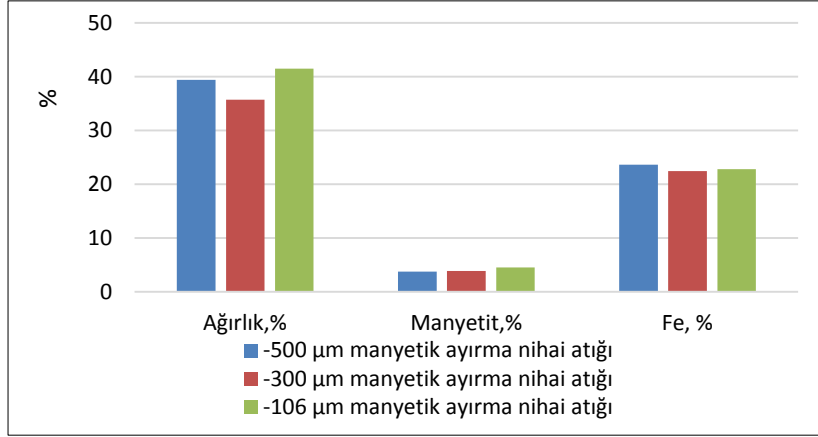
Şekil 9. Tüm tane boylarında, beslemedeki toplam manyetitin atıklara dağılımı.
