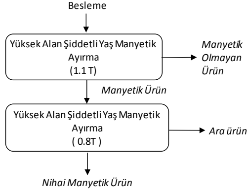
Şekil 5. Atığa uygulanan yüksek alan şiddetli yaş manyetik ayırma işlemi test şeması. Figure 5. High-gradient wet magnetic separation test procedure applied to waste.
