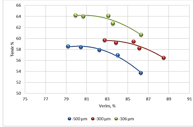
Şekil 10. Farklı inceliklerde manyetik ayırma testi tenör-verim ilişkisi.
