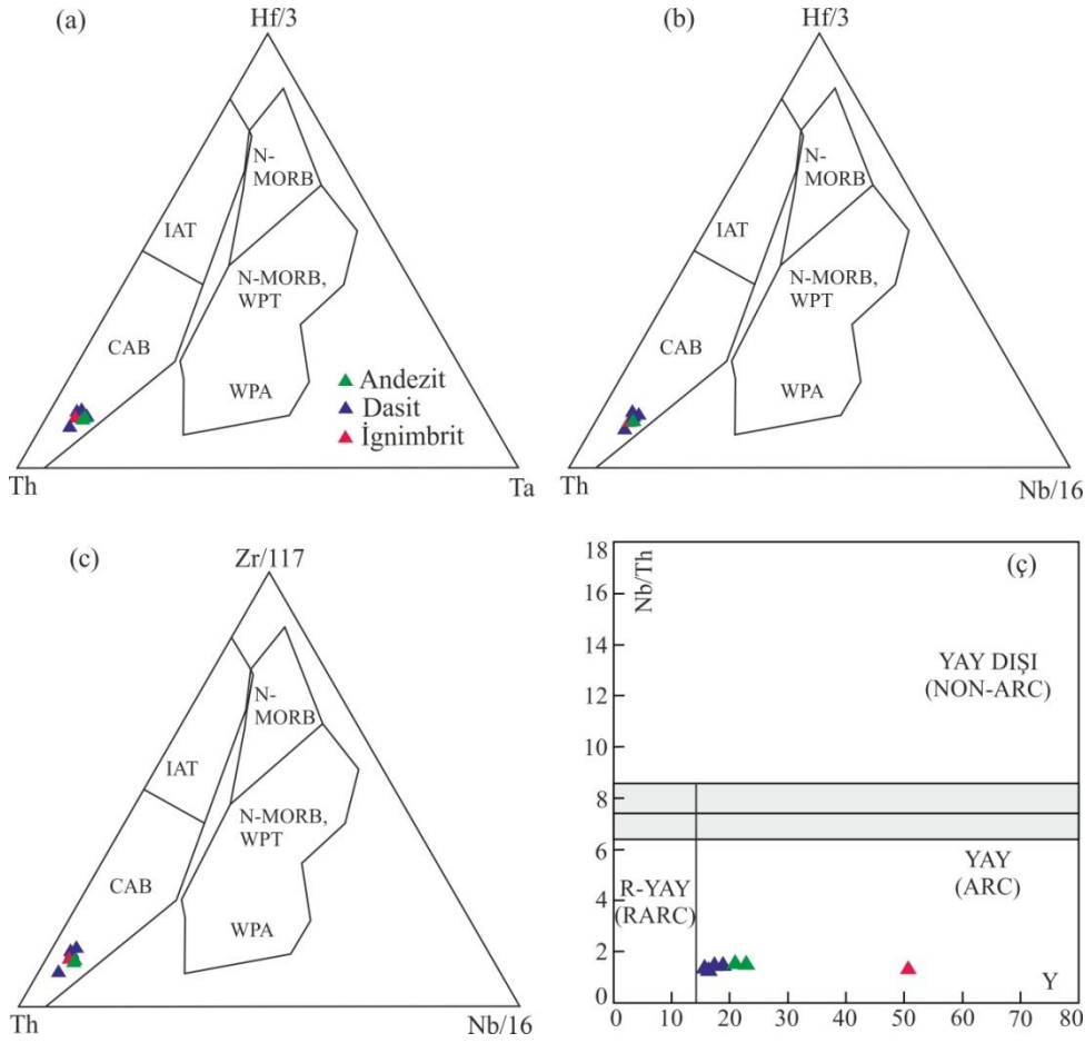
Şekil 9. a-b-c) Vulkanik birimlere ait Wood (1980)'e göre yapılmış tektonik ayırtlama diyagramları (Th-Hf-Ta-Zr-Nb) (CAB: Kalk-alkali yay bazaltları, IAT: Ada yayı toleyitleri, N-MORB: Normal okyanus ortası sırt bazaltları, E-MORB: Zenginleşmiş okyanus ortası sırt bazaltları, WPT: Levha içi toleyitleri, WPA: Levha içi alkali), ç) Nb/Th'a karşı Y tektonik ayırtlama diagram (Swinden et al., 1990) (RARC: Refrakter yay volkanik alanı).
