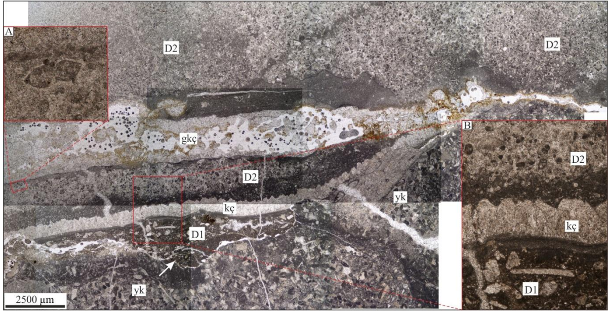
Şekil 6. D1 ve D2 dolgularını ve yan kayaç ilişkilerini gösteren ince kesit fotoğrafı (örnek no: 03-618). Yan kayaç (yk) baskın olarak yıkanmış biyoklastik Tanetaşı dokusuna sahiptir. İstiftteki olasılıkla en yaşlı dolgu olan D1 dolgusu köşeli allokemlerin (olasılıkla biyoklast) mikrit içinde yüzdüğü bir dokuya sahiptir ve yan kayaç ile düz olmayan bir sınır ilişkisi sunar (ok). D1 dolgusu ve yan kayaç kalsit çimento (kç) ile kaplanmış ikinci bir dolgu yüzeyi tarafından kesilmiştir. Kalsit çimentonun çökelinein ardından ikinci nesil dolgu (D2) gerçekleşmiştir. D2 dolgusu seyrek planktonik foraminifer, kalsisifer ve tanımlanamayan biyoklastlar içeren Vaketaşı/Çamurtaşı dokusu ile temsil edilir. Tüm doku kalsit dolgulu genç bir çatlak (gkç) tarafından kesilmektedir. A) D2 dolgusu içerisinde gözlenen dicarinellid ( D. aff. primitiva )'in yakından görünümü, B) D1 ve D2 dolguları ile iki dolgu arasında gözlenen kalsit çimentonun (kç) ayrıntısı.
