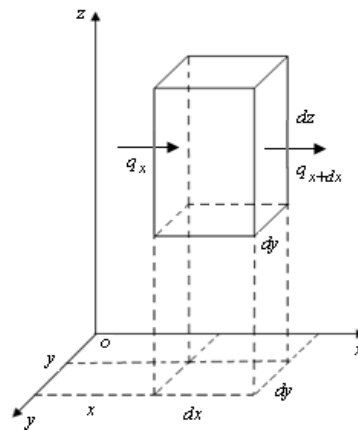
Şekil 3. Küçük (Elementer) hacimden geçen ısı akımı
