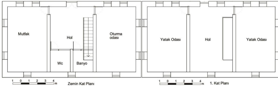
Şekil 2. Bağ evinin zemin katı.
