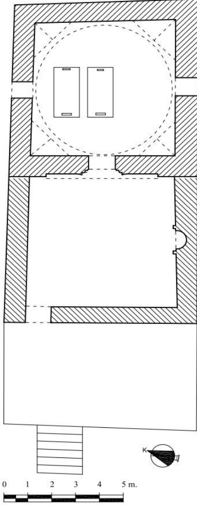
Çizim 1: Havsa Hatun Türbesi Planı
