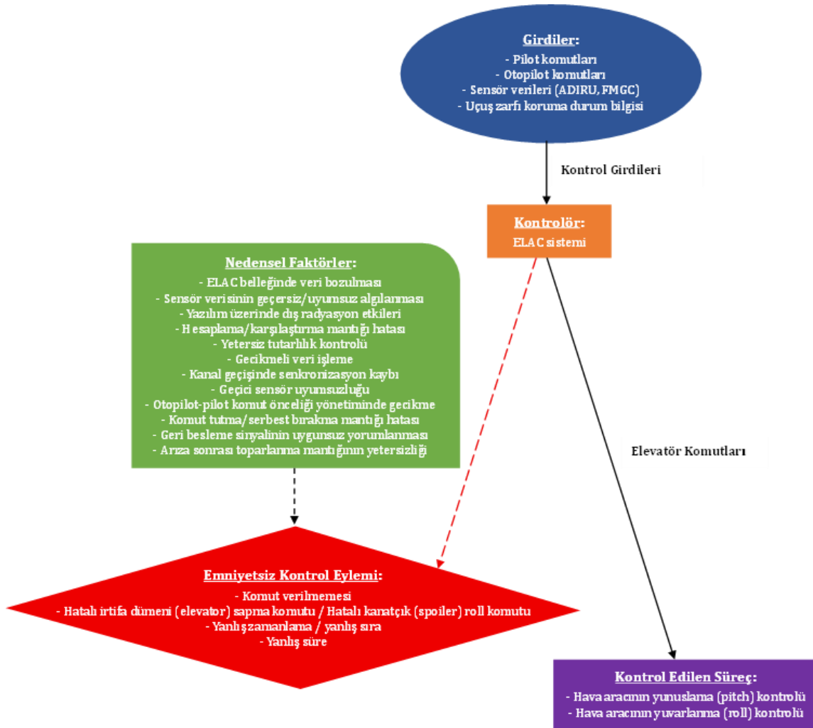
Şekil 4. ELAC'ın pilot girdileri, kontrol yüzeyleri ve geri bildirimle nasıl etkileştiğini gösteren STPA temelli kontrol yapısı.
