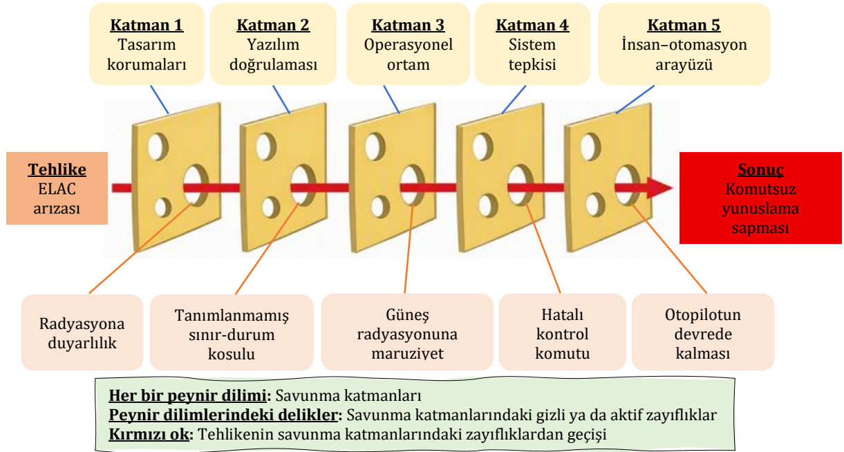
Şekil 5. Hizalanmış gizli veya aktif zayıflıkların ELAC ile ilişkili yunuslama sapması olayına nasıl yol açtığını gösteren İsviçre Peyniri modeli.
