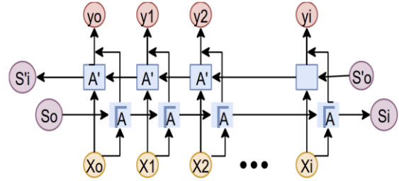
Şekil 10. Bi-LSTM'nin blok şeması (Kaysal vd., 2023).
