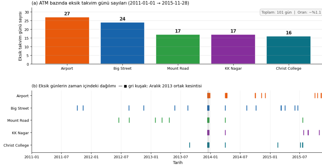
Şekil 6. Kullanılan dönemdeki (2011-01-01 – 2015-11-28) eksik takvim günlerinin ATM bazında dağılımı. (a) Her ATM için toplam eksik gün sayısı; (b) eksik günlerin zaman içindeki dağılımı.
