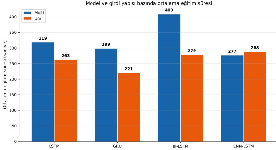
Şekil 14. Model ve girdi yapısı bazında ortalama eğitim süresi (saniye).
