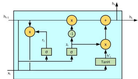
Şekil 8. GRU mimarisi (Tosun ve Şentürk, 2023).
