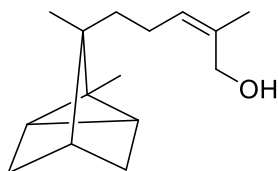
\alpha -Santalol
