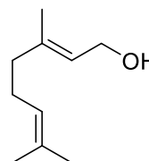
Geraniol
