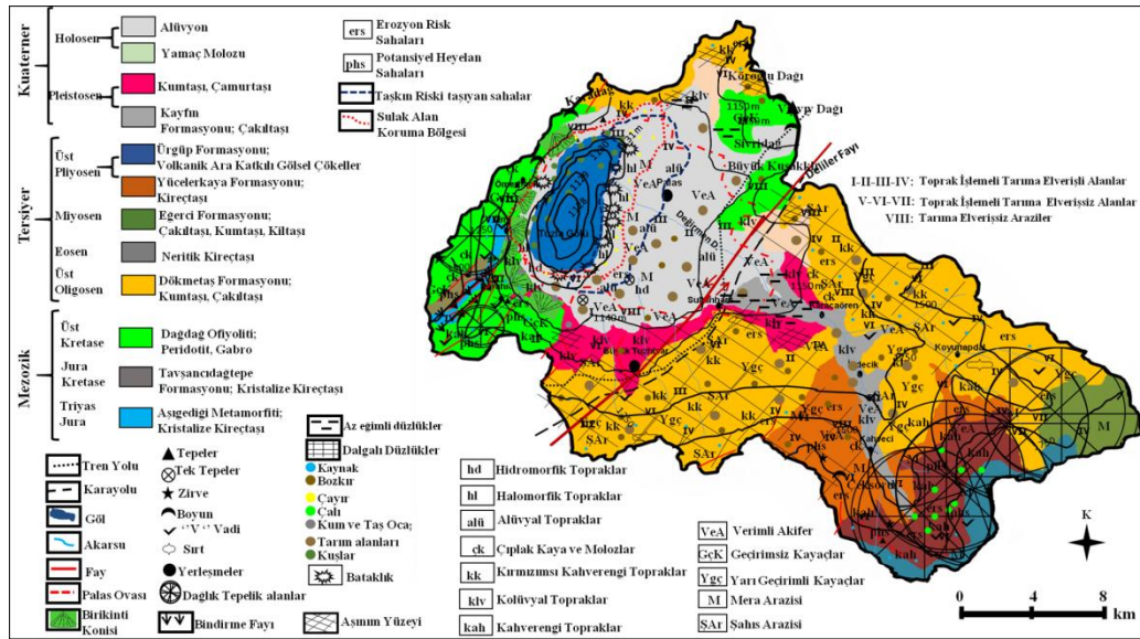
Şekil 2: Çalışma Sahasının Uygulamalı Jeomorfoloji Haritası
