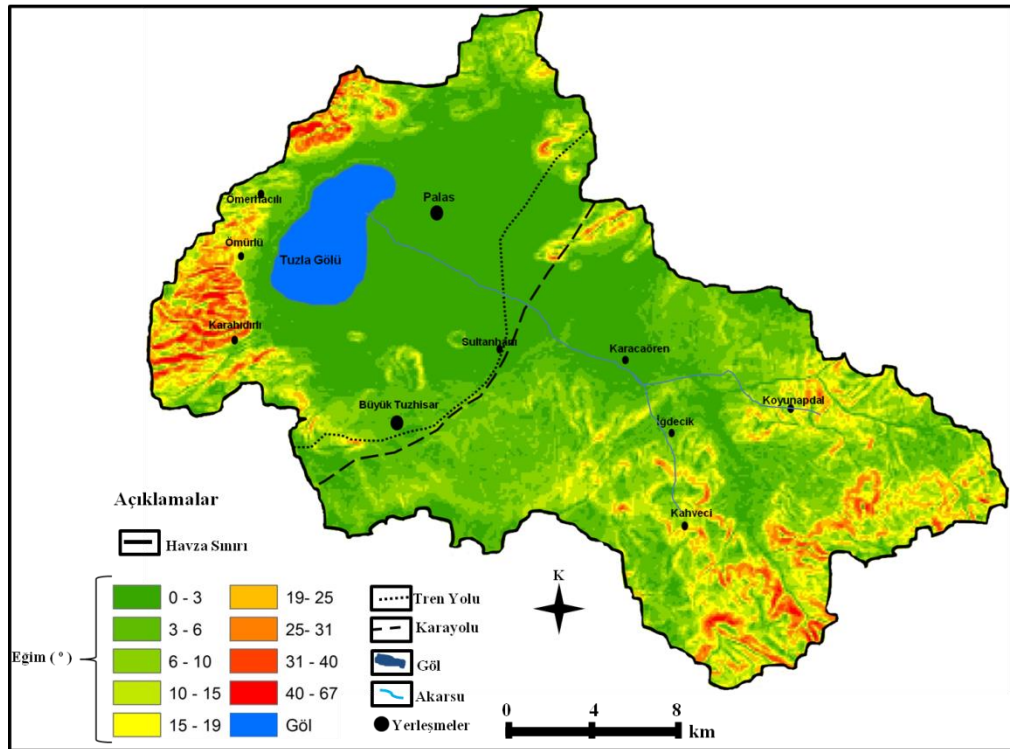
Şekil 4: Çalışma Sahasının Eğim Haritası
