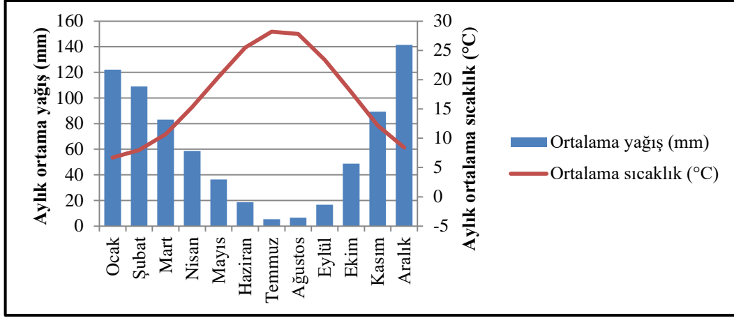
Şekil 3: Manisa Uzun Yıllık Ortalama Sıcaklık-Yağış Grafiği (1960-2016)
