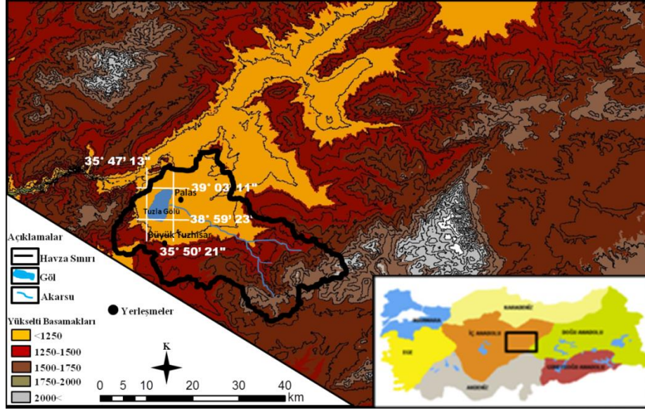
Şekil 1: Tuzla Gölü Havzası Lokasyon Haritası
