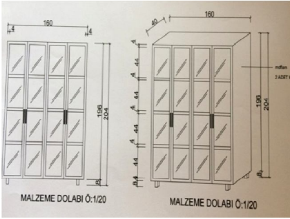
Şekil 10. Malzeme Dolabı Planı.
