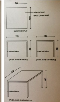
Şekil 7. Çalışma Masaları Planı
