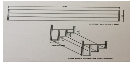
Şekil 14. Kurutma Alanı ve Askılık Planı.
