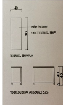
Şekil 8. Tekerlekli Sehpa Planı
