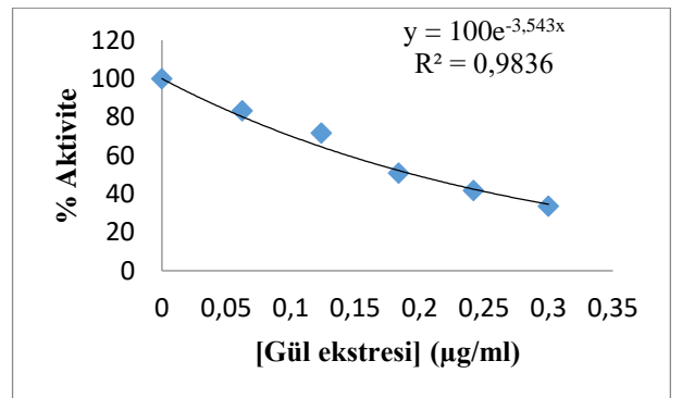
Şekil 2. Gül suyu ile BChE IC 50 grafiği.
