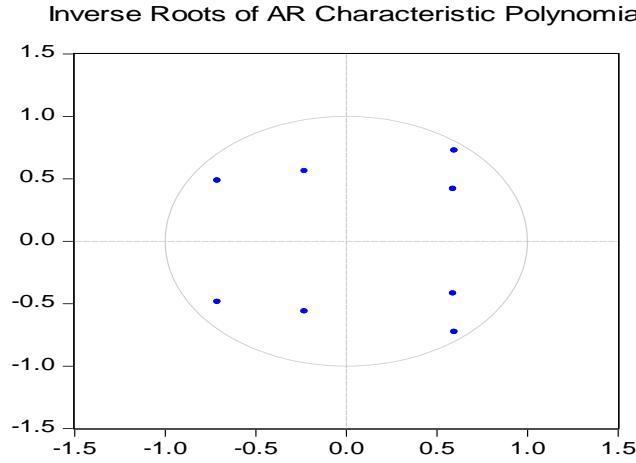
Grafik 6: Ar Karakteristik Polinomunun Ters Köklerinin Birim Çember İçindeki Konumu
