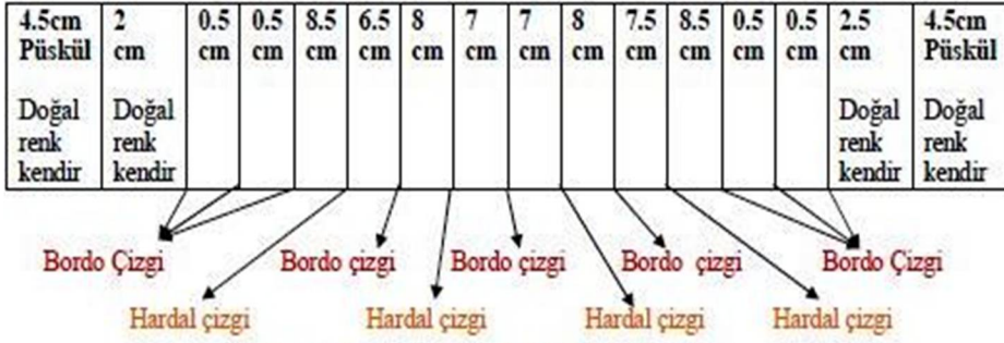
Çizim 13. Emriye Bilgin'in Dokuduğu Peşkir Teknik Çizimi
