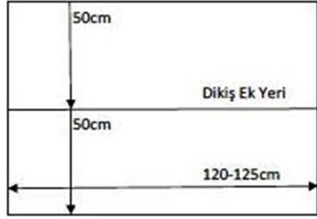
Çizim 7. Şal peştamal Teknik Çizimi
