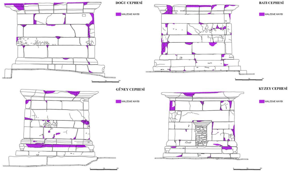
Fig. 5: Cephelerde yapılan malzeme kaybı haritaları.
