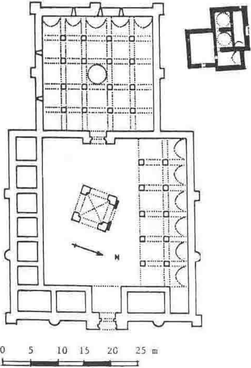
Çizim 4: Afyon-İshaklı Sâhib Ata Kervansarayı ve Hamamının Planları (H.Karpuz'dan)
