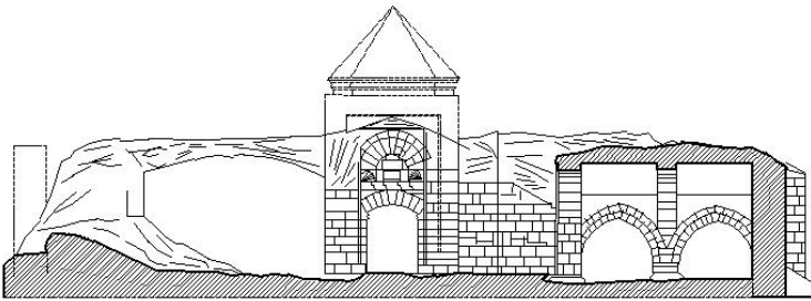
Afyon-İshaklı Sâhib Ata Kervansarayı Kesiti (E.İ.İ. Abd. Yp. İş.Dai. Bşk.Arşivi'nden Düzeltildi)
