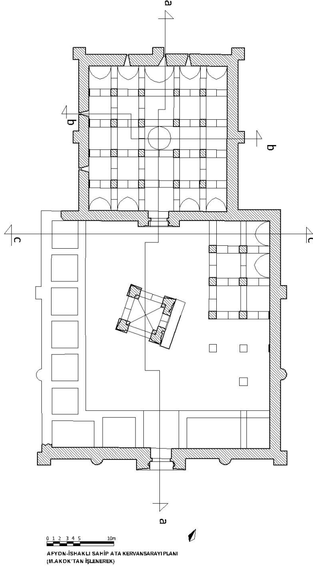
Çizim 1: Afyon-İshaklı Sâhib Ata Kervansarayı (Onarım Öncesi) Planı (Akok'tan İşlenerek)
