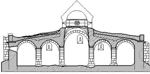
Afyon-İshaklı Sâhib Ata Kervansarayı Kesiti (E.İ.İ. Abd. Yp. İş.Dai. Bşk.Arşivi'nden Düzeltildi)
