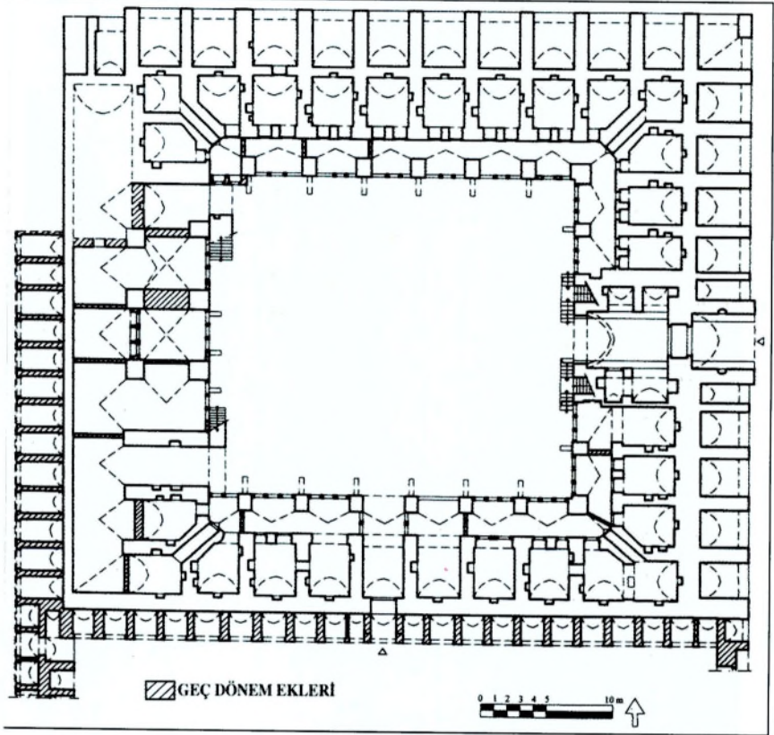
Plan 1 - Gümrük Hanı alt kat rölöve planı.
