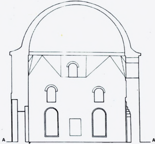
Şekil 2. Edirne- Karaağaç Timurtaş Köyü Timurtaş Paşa Camisi'nin A- A kesiti
