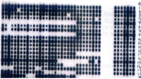
Resim 1 : MTBK izolatlarının spoligotipleme görüntüsü
