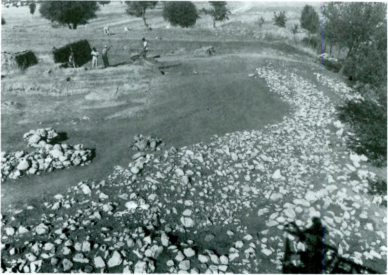
Levha 36/2 - İTÇ'nin yamaç döşemesi -glacis-.
