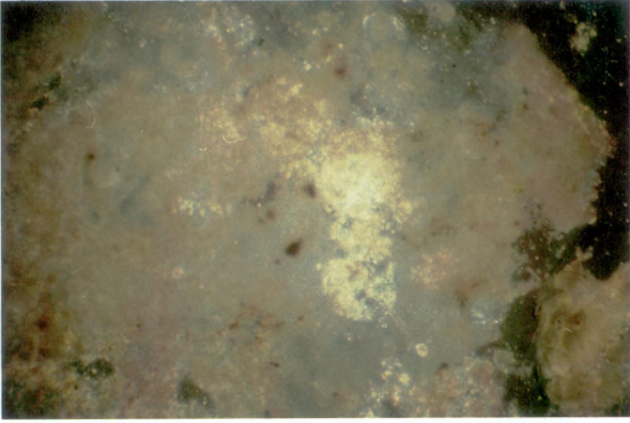
Levha 51/1 - Kripto (kil boyutlu) kristalli bağlayıcı kireç hamuru ortasında nispeten iri kristaller.
