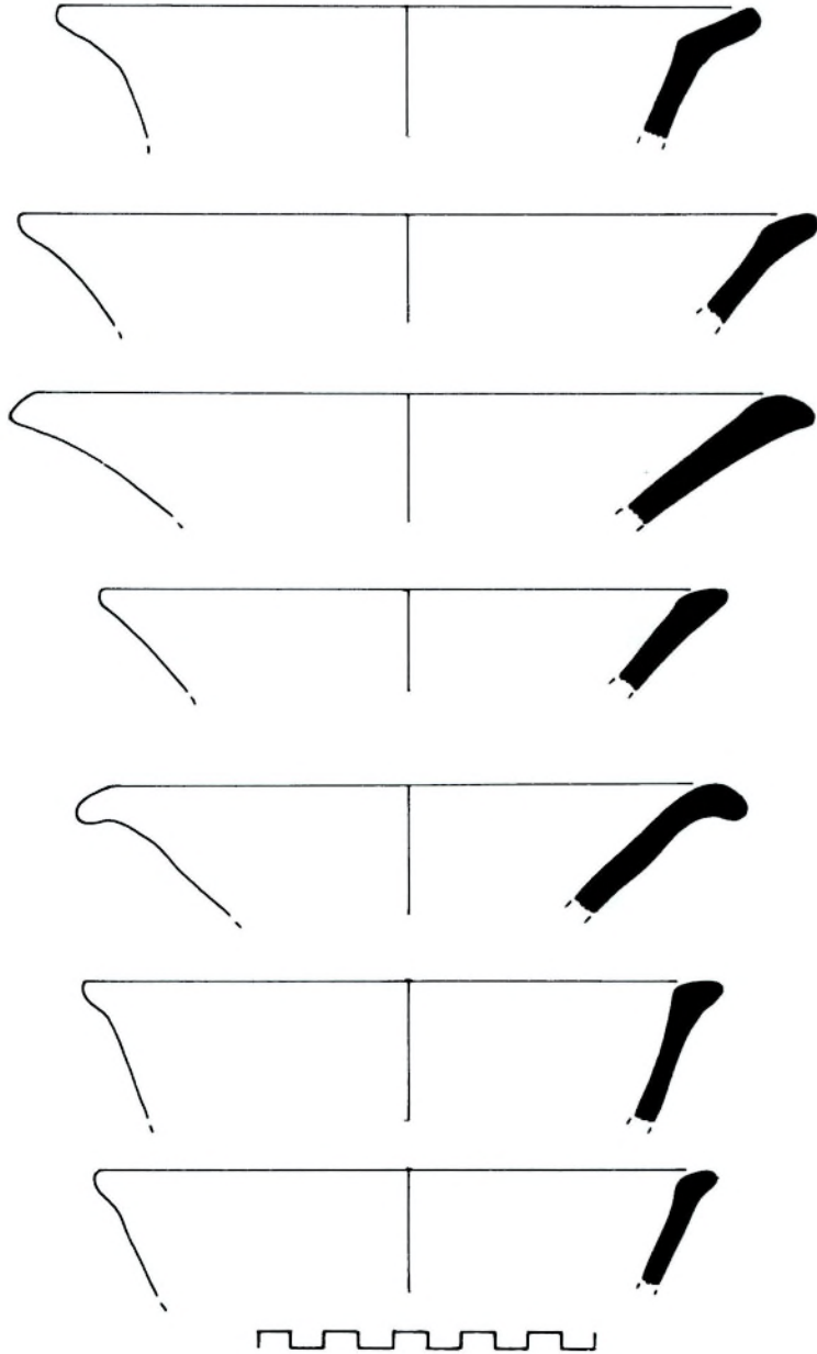
Levha 20 - 'Izgara Temeller'in yakınlarında bulunan çanak çömleğinden örnekler.
