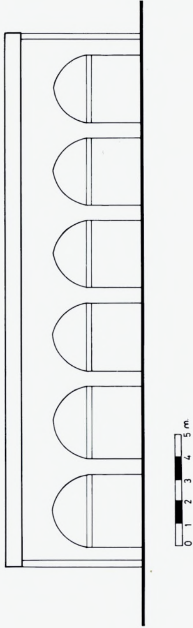
Çizim 6 - Bor Sokullu Mehmet Paşa Arastası, boyuna kesit.
